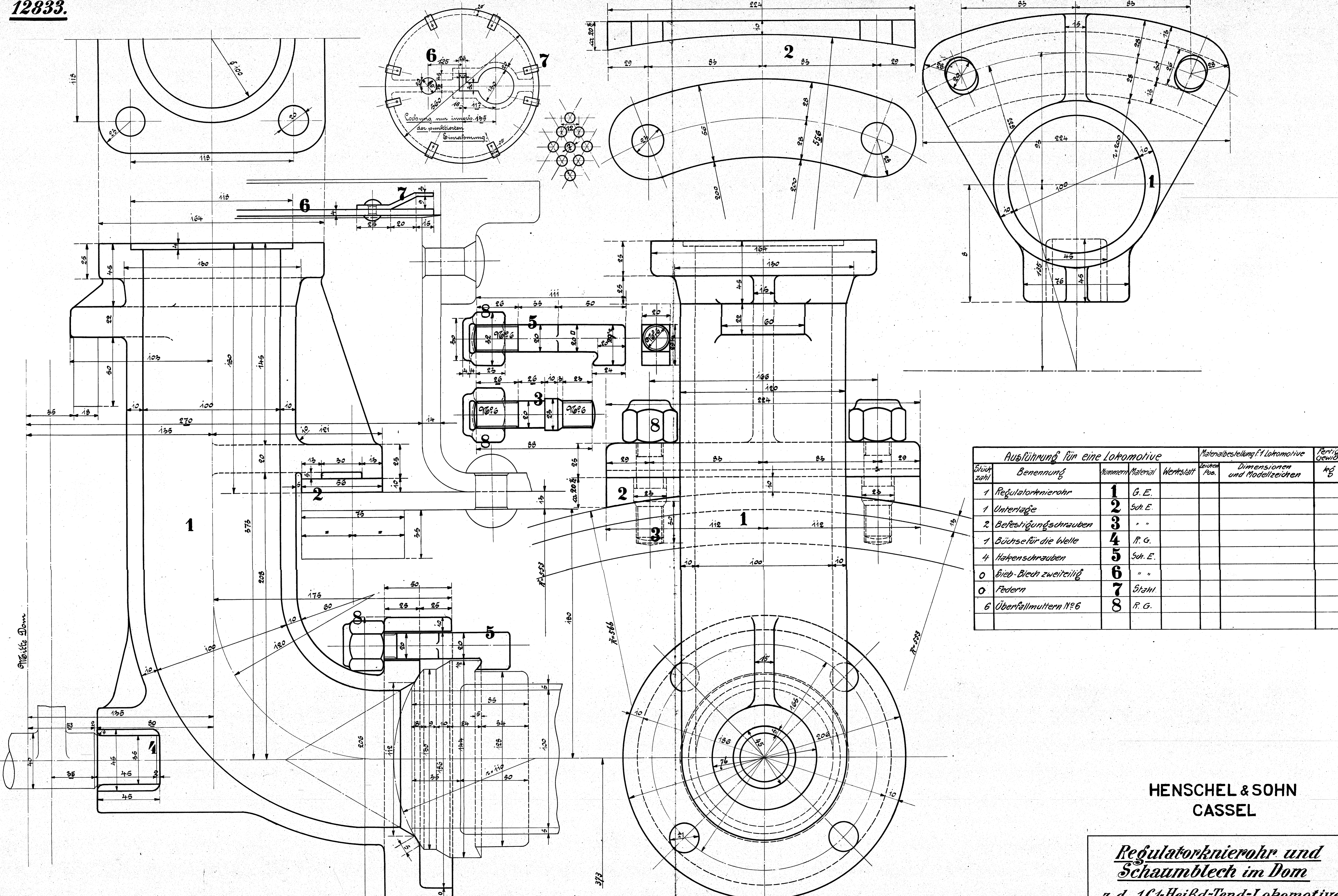
Regulatorknierrohr u. Schaumblech im Dom.
