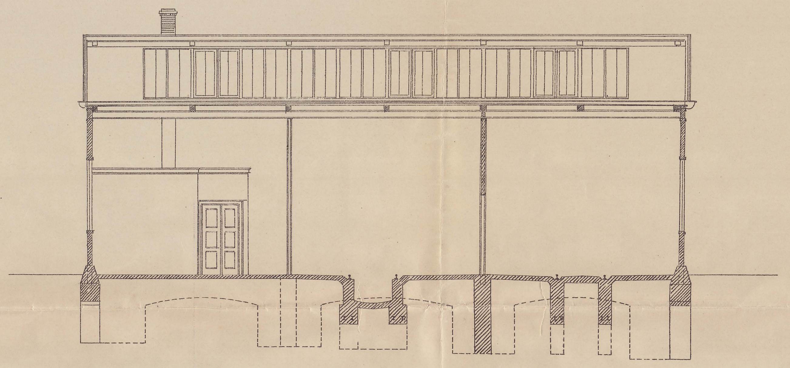
SNIT A-B.
