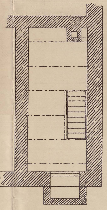
KÆLDERPLAN.
