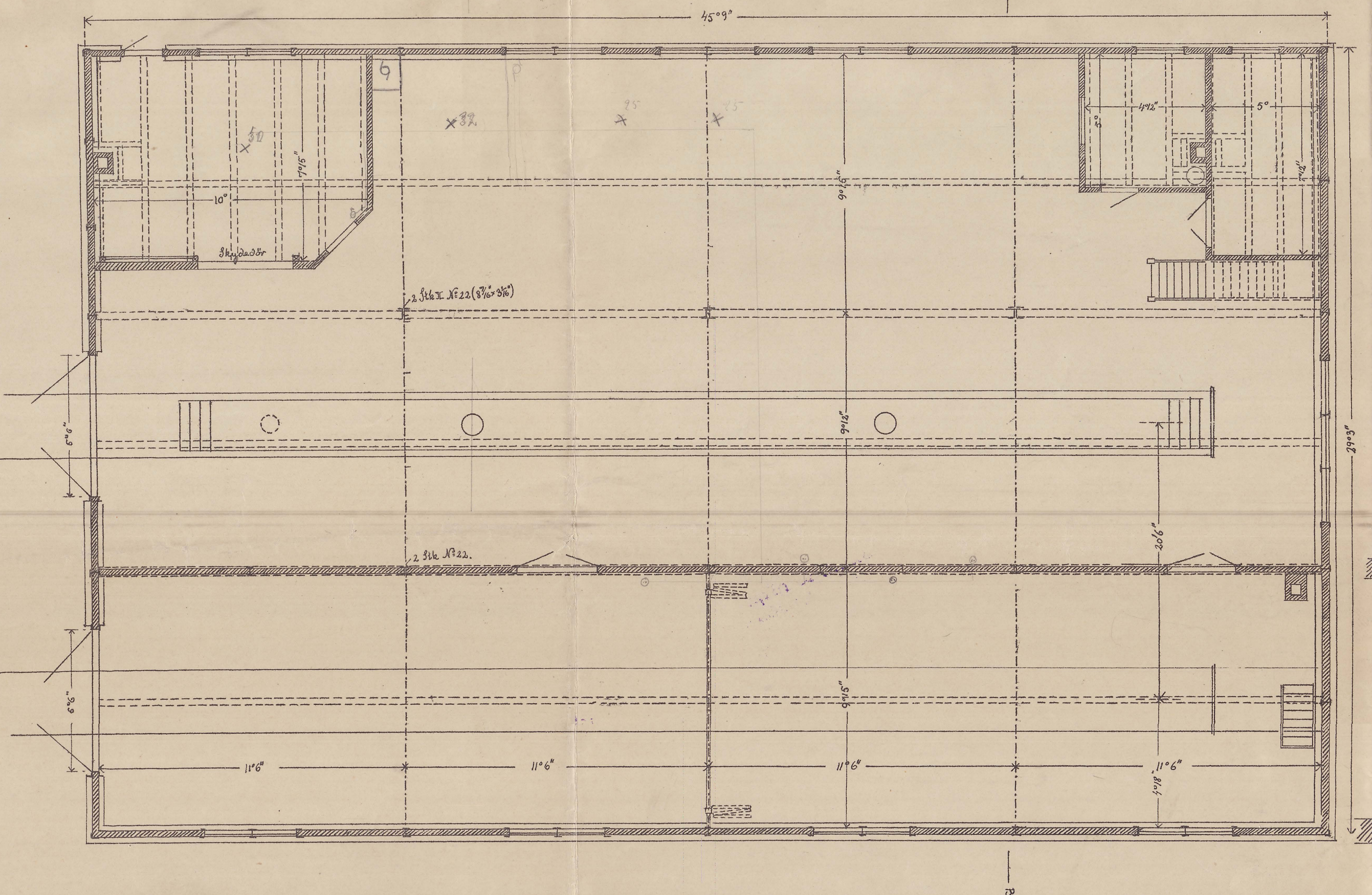
KÆLDERPLAN.
