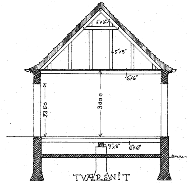
TVÆRSNIT
