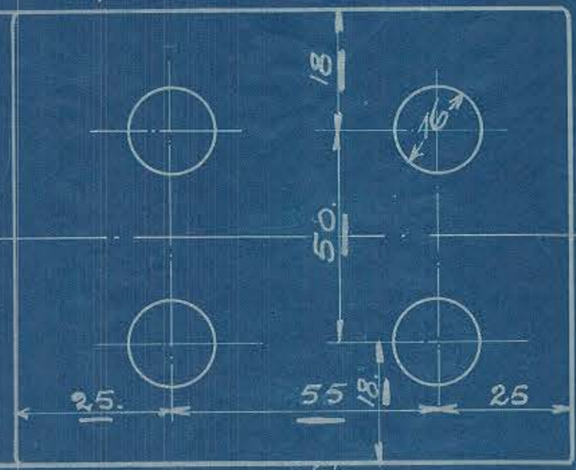
FÖR I-LÅNGBALK.
