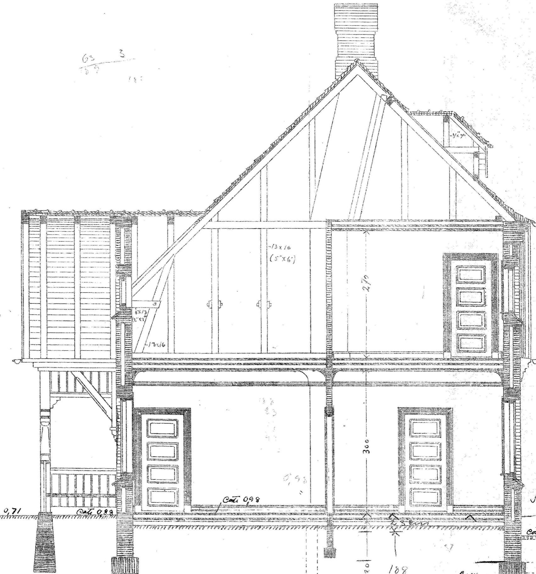
SNIT.
