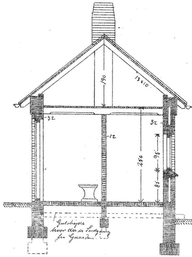
SNIT.
