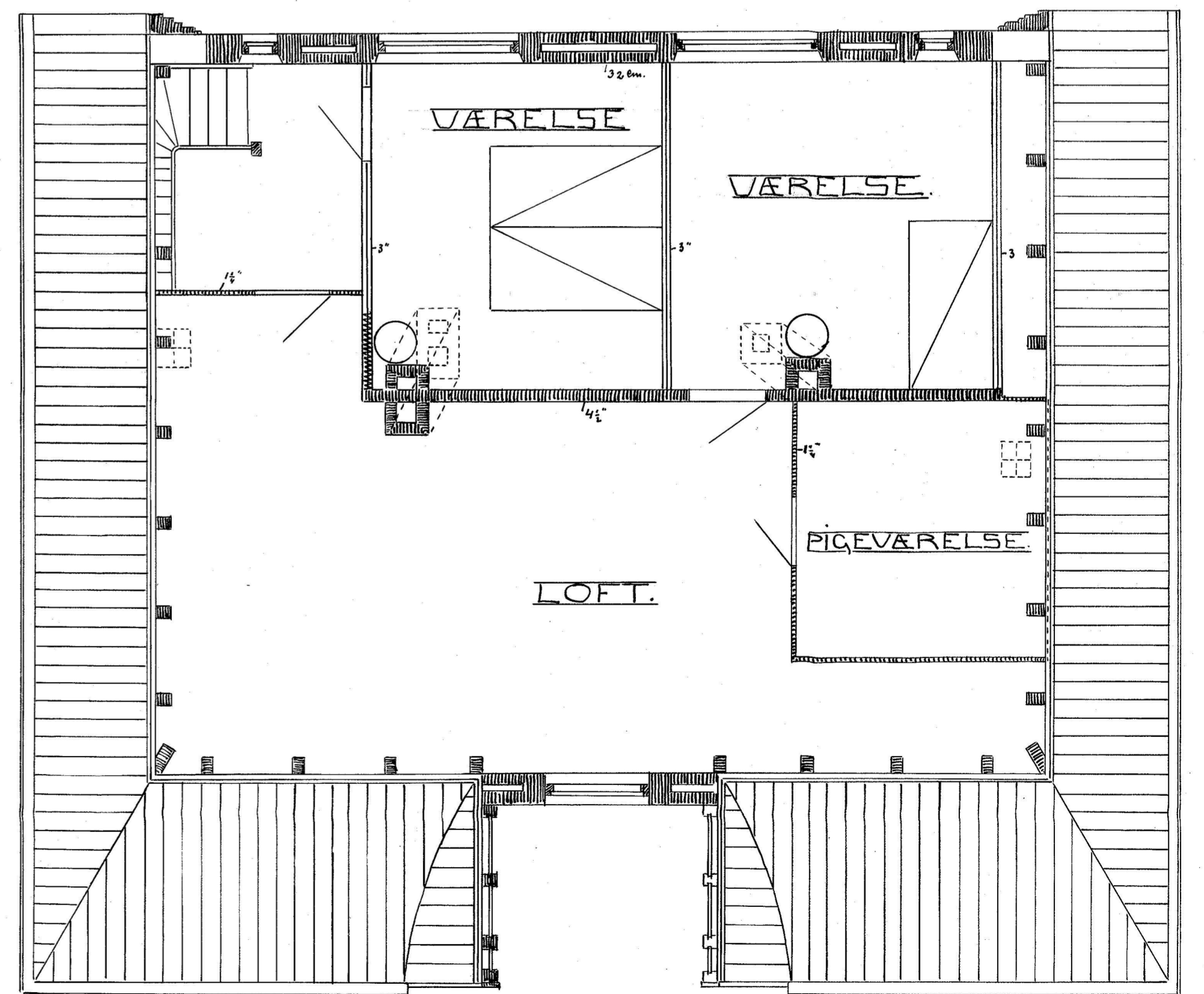
LOFTSPLAN.
