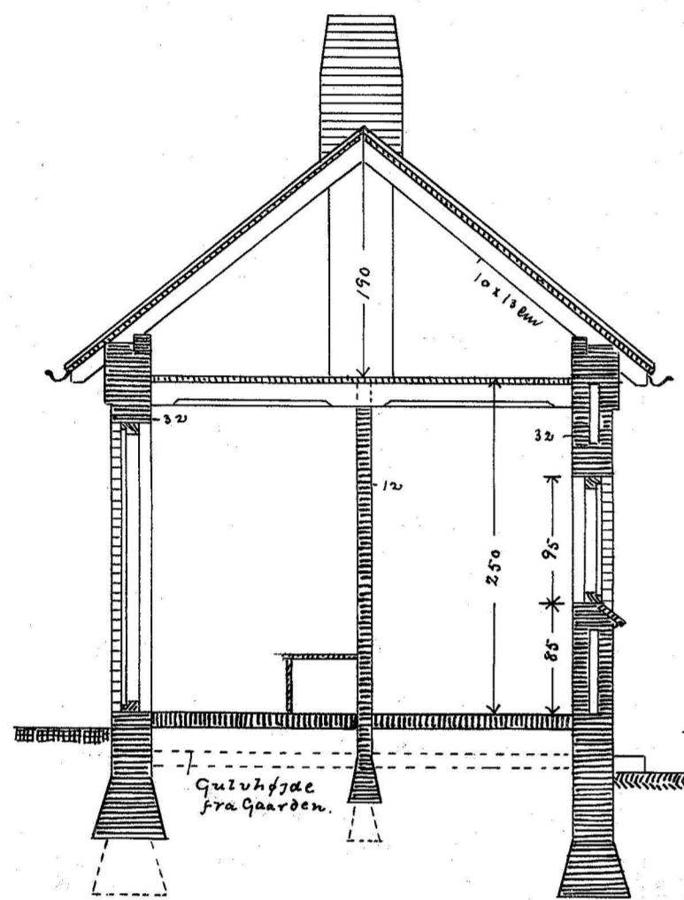
SNIT.
