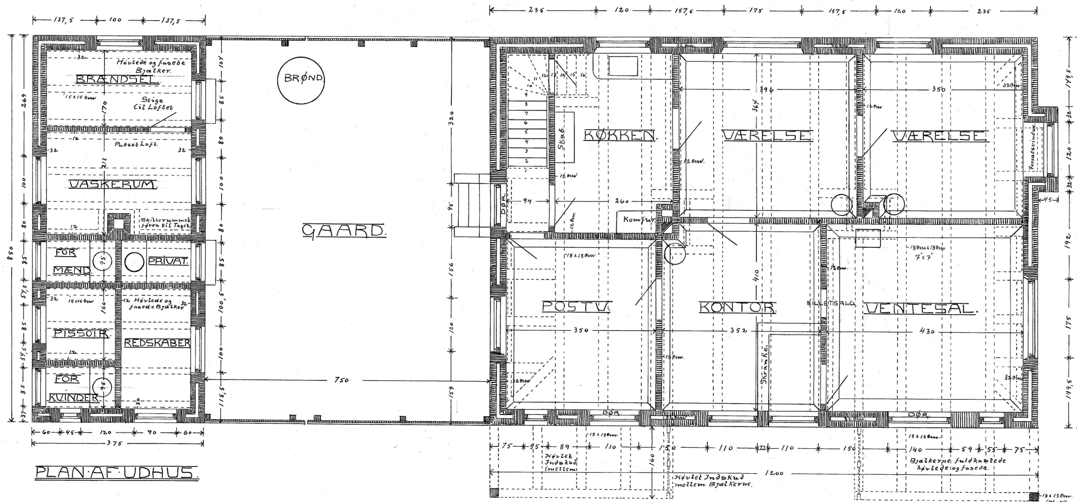
STUEPLAN.
