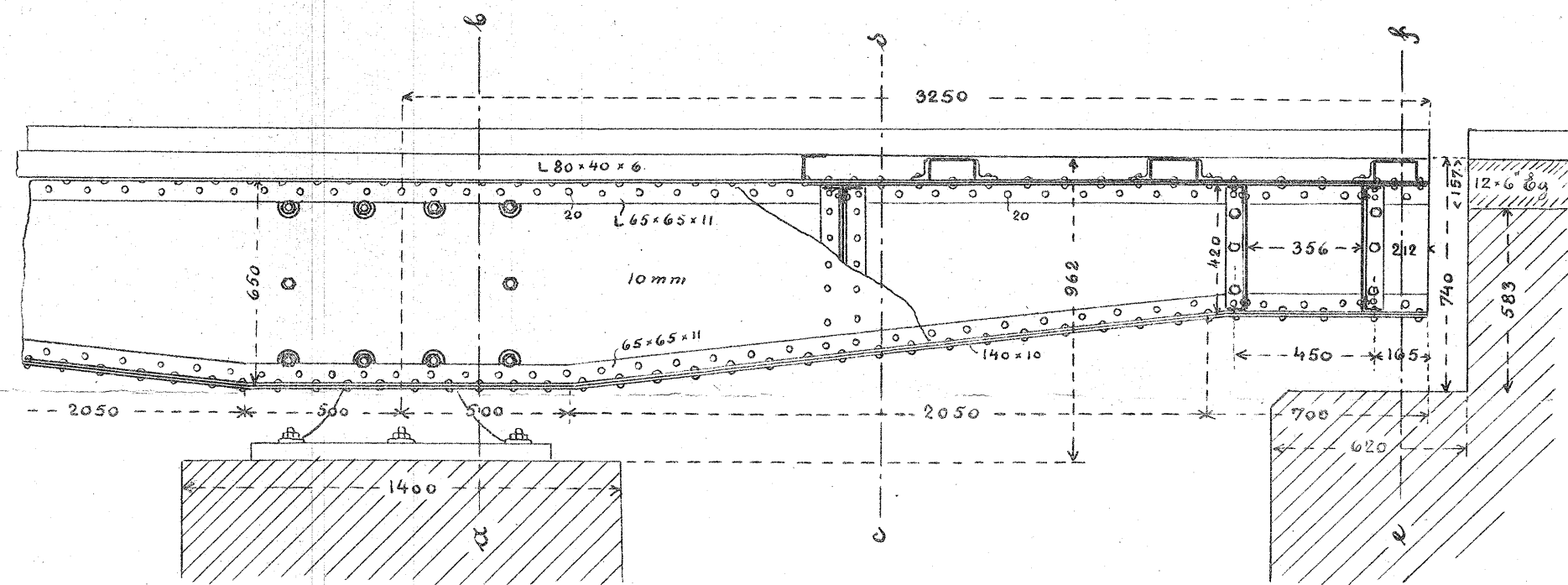
Længdesnit g-h.
