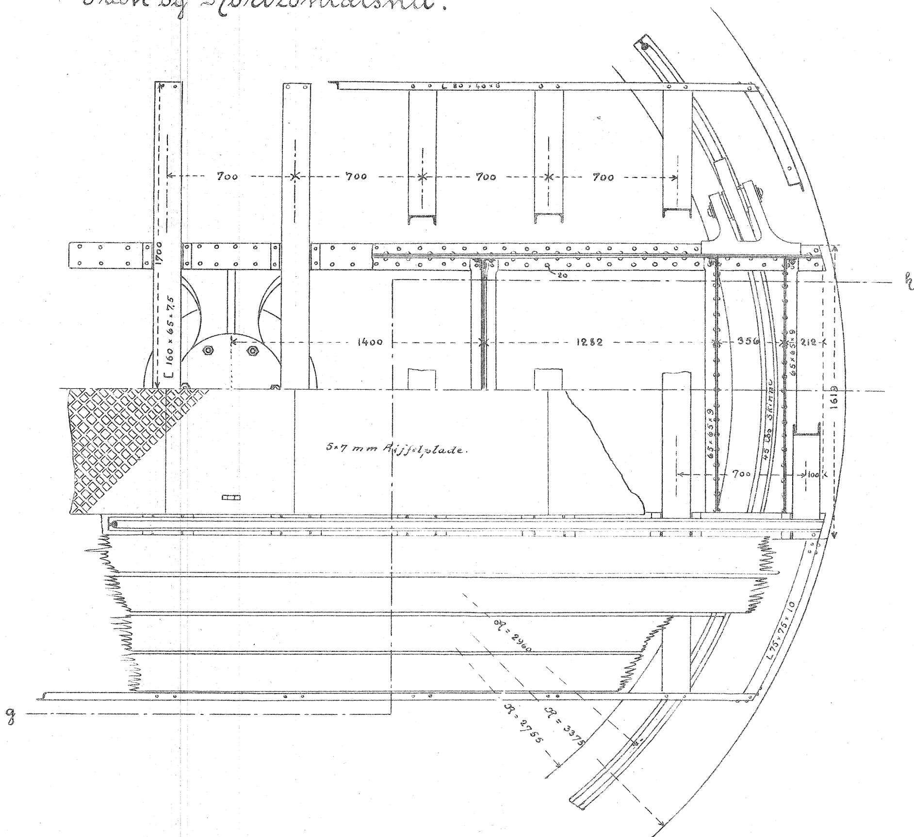
Plan og Horizontalsnit.
