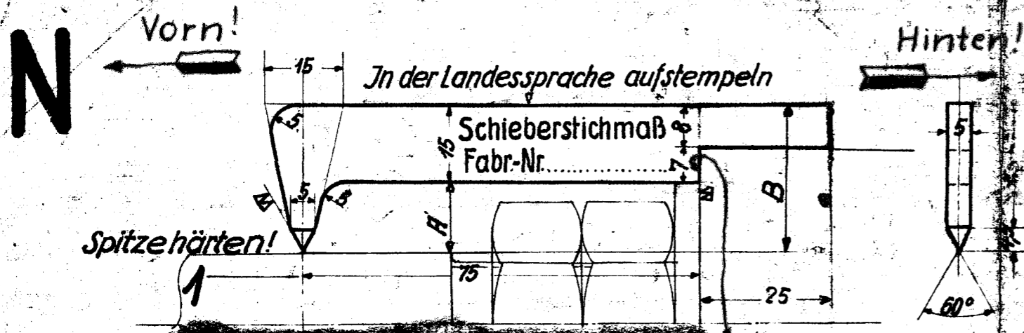
Vorderkante Pos 13. Schieberstangenkreuzkopf Zeichng. 2124
