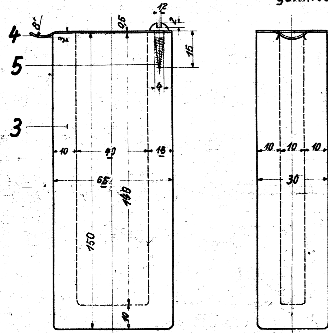
Vorderkante Pos 13. Schieberstangenkreuzkopf Zeichng. 2124
