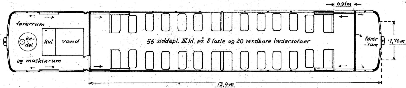
Rekonstruktion efter fotos, brochurer samt opmåling af passagerdelen, der endnu ligger som glasveranda i Helsingør maj 1974. A. Hkjær
