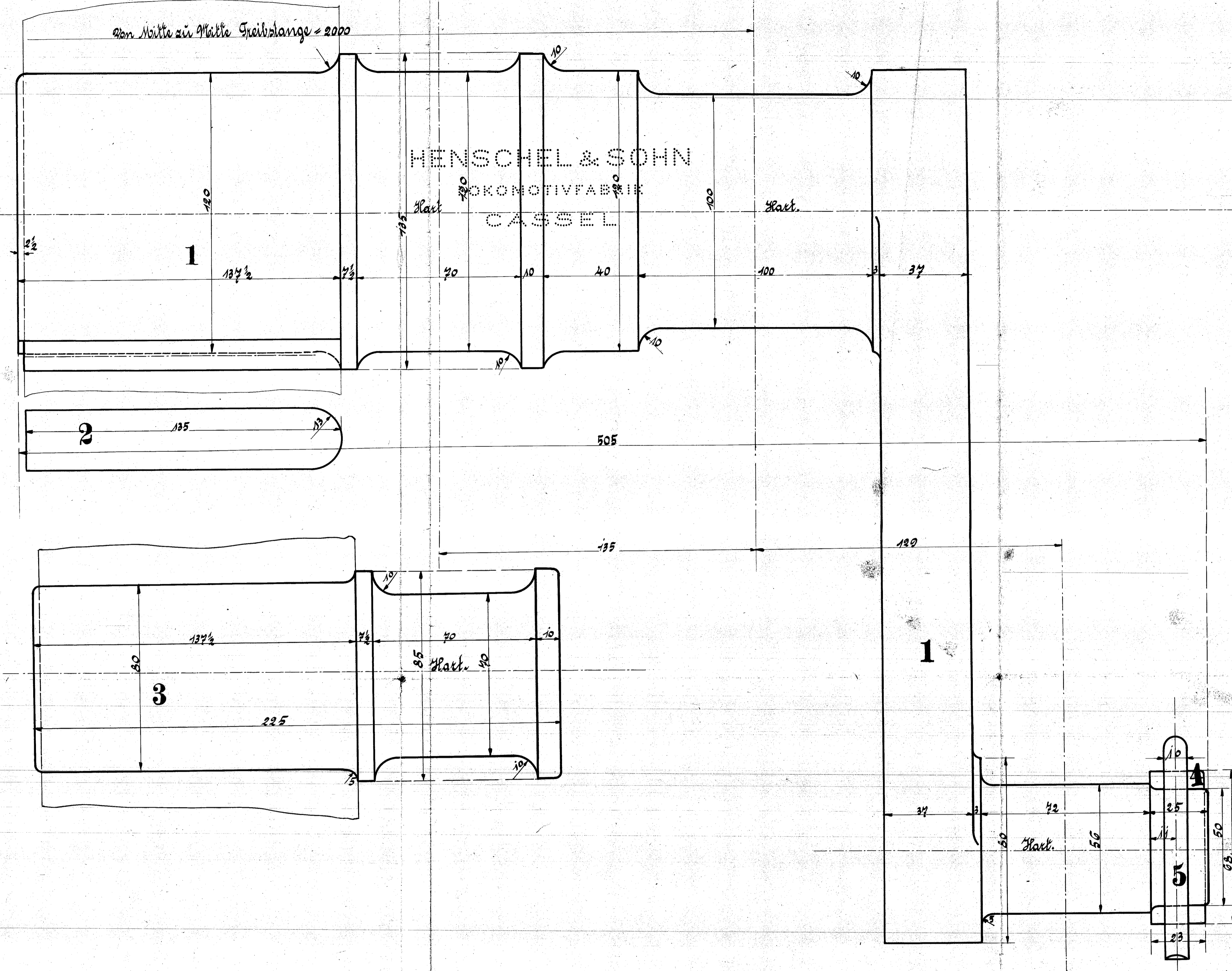
Einrichtung für 1 Lokomotive
