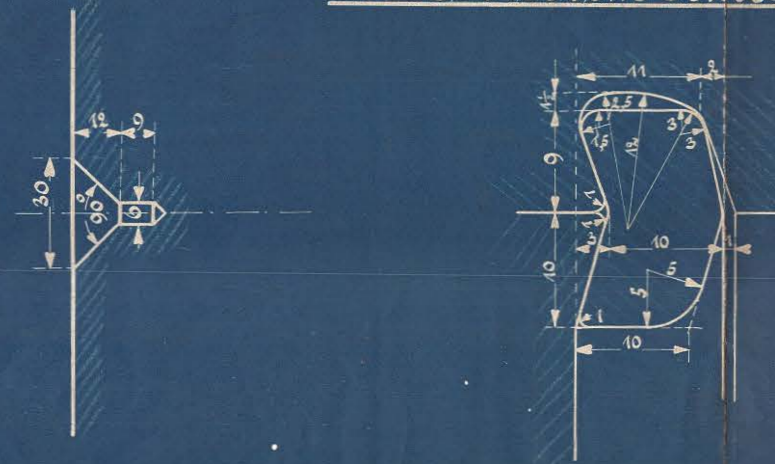
Querschnitt des Sprengringes und der Nut vor dem Oetreiben.
