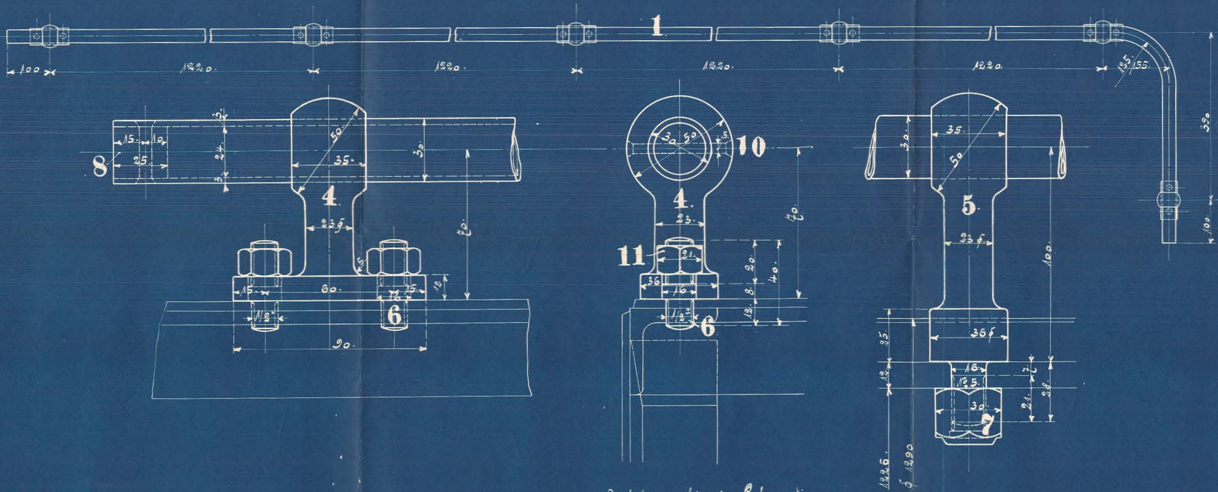
Anschluß für eine Lokomotive.
