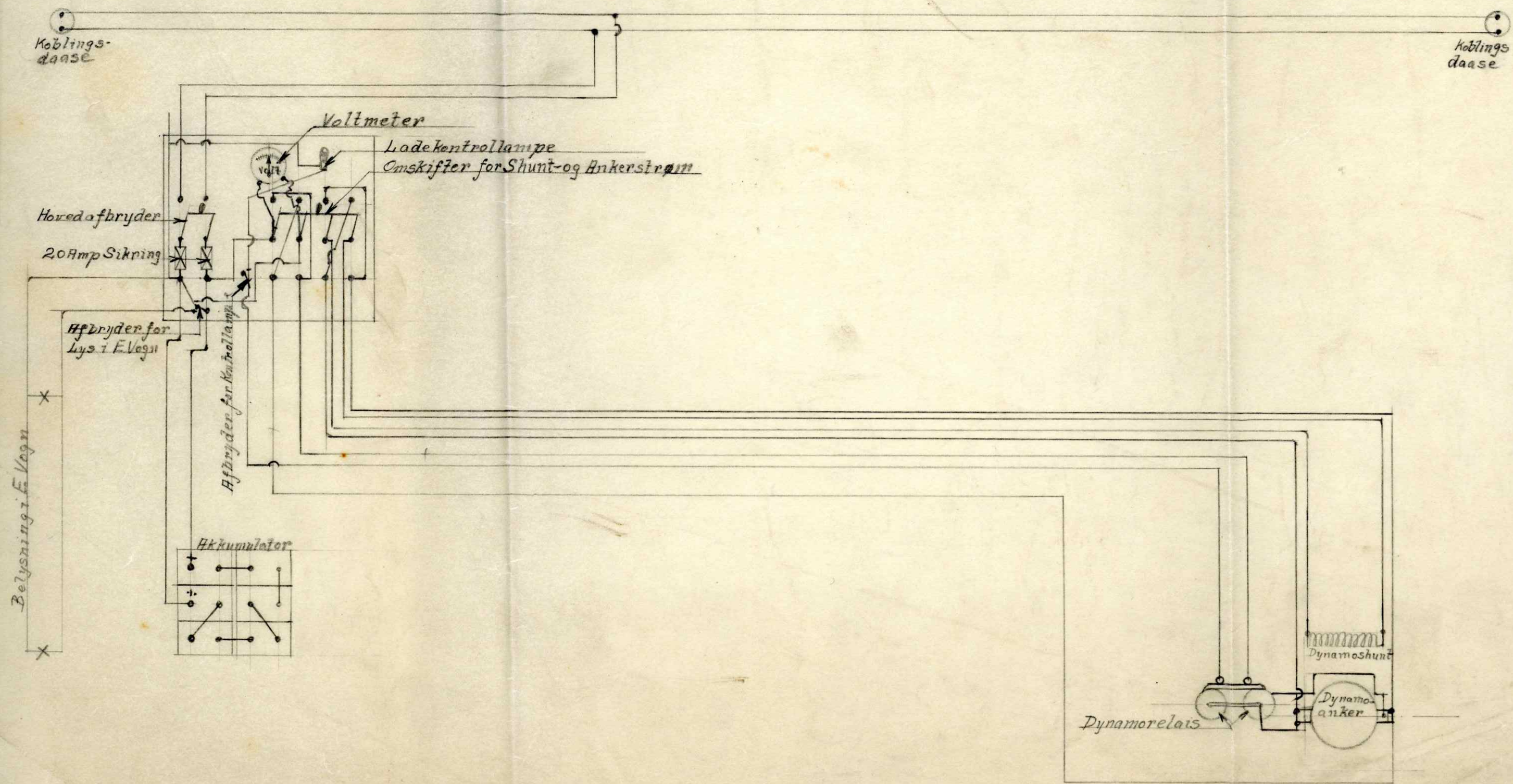
Strømskema for Anlæg i E161
