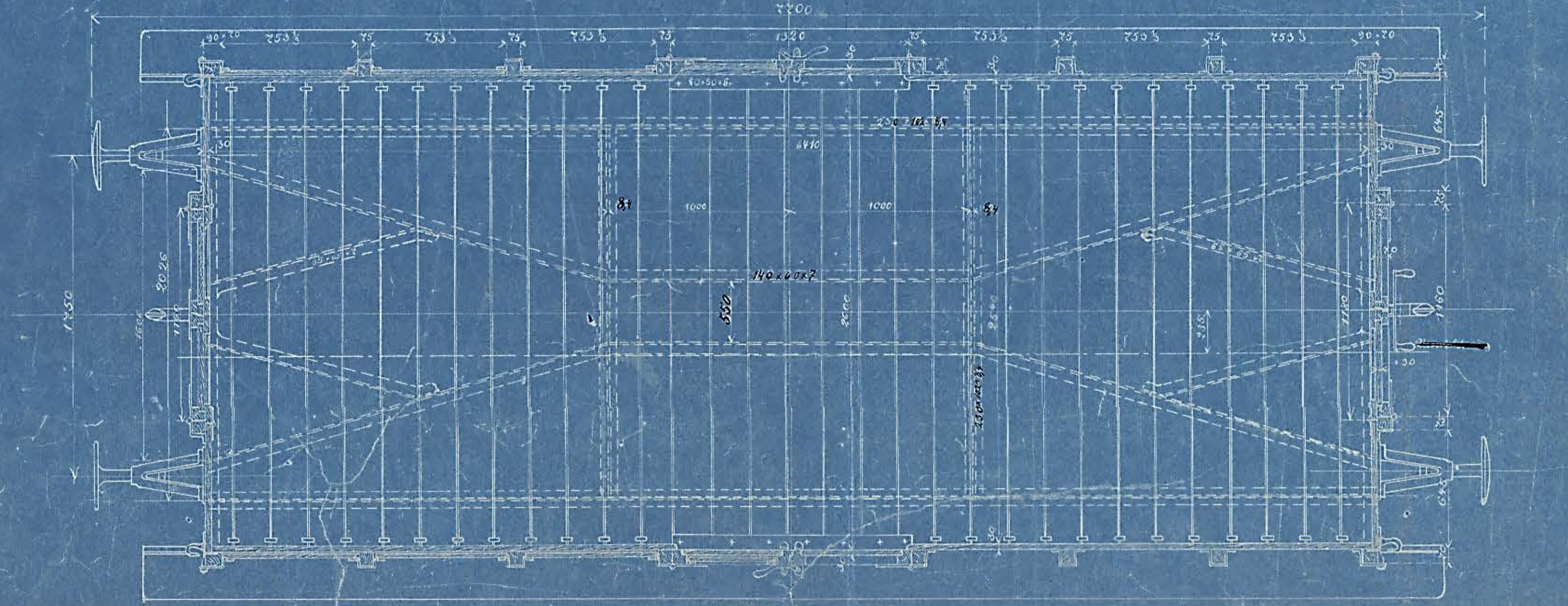
Lukket Godsvoagn med Haandbremse til Nordjyllands forenede Privatbaner.
