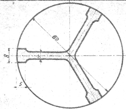
Querschnitt des Sicherheitsventils in natürlicher Größe
