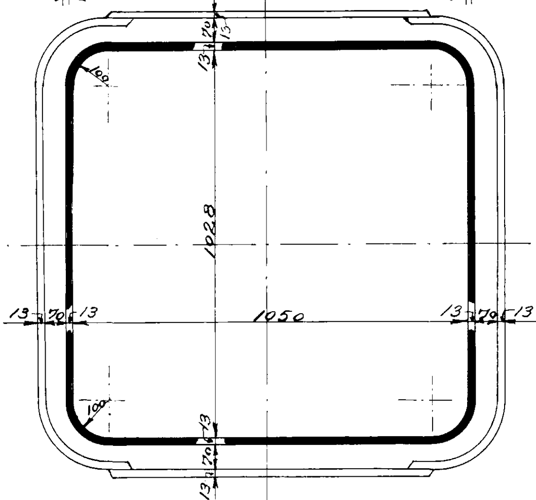
Kobber-Fyrkasse Loko. Type II a.
