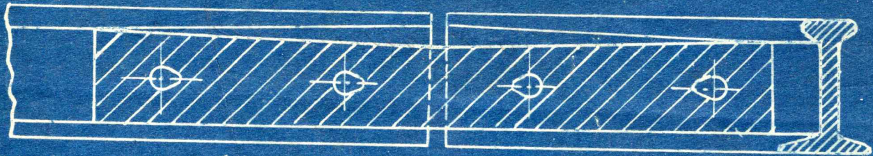
Ausgeschlagene Laschenkammer und Lasche.
