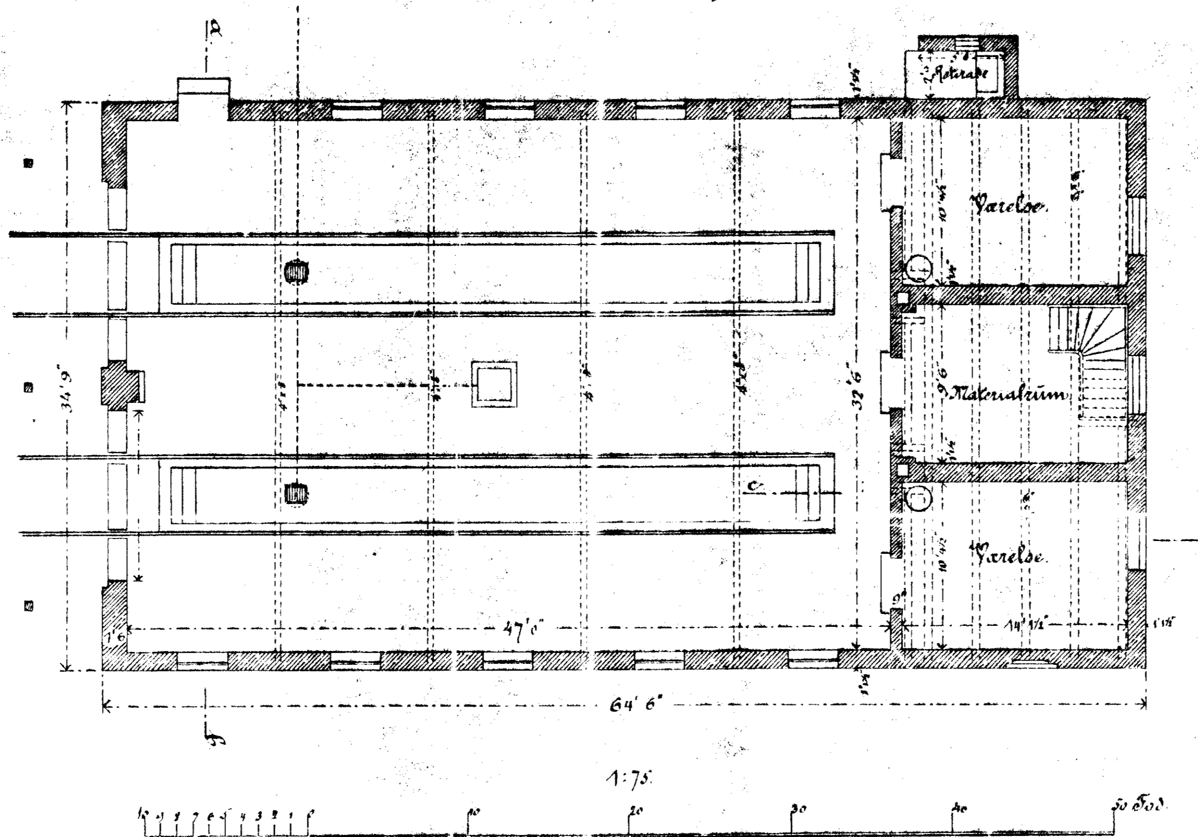
Snit af 1. etagen.
