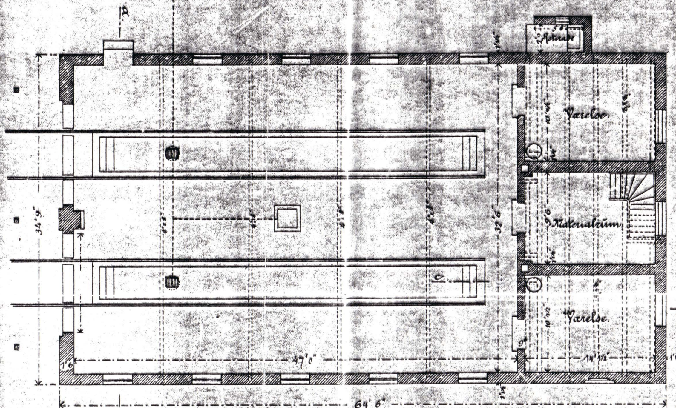
Plan af 1. etagen.
