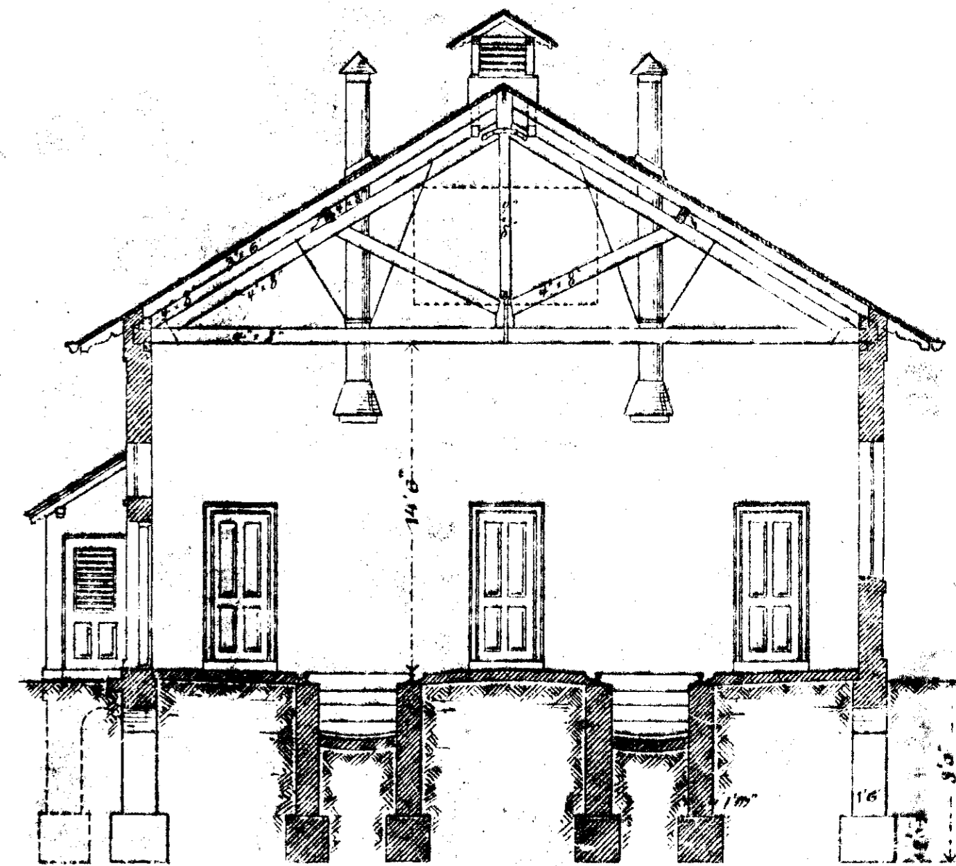
Snit af 2. etagen.
