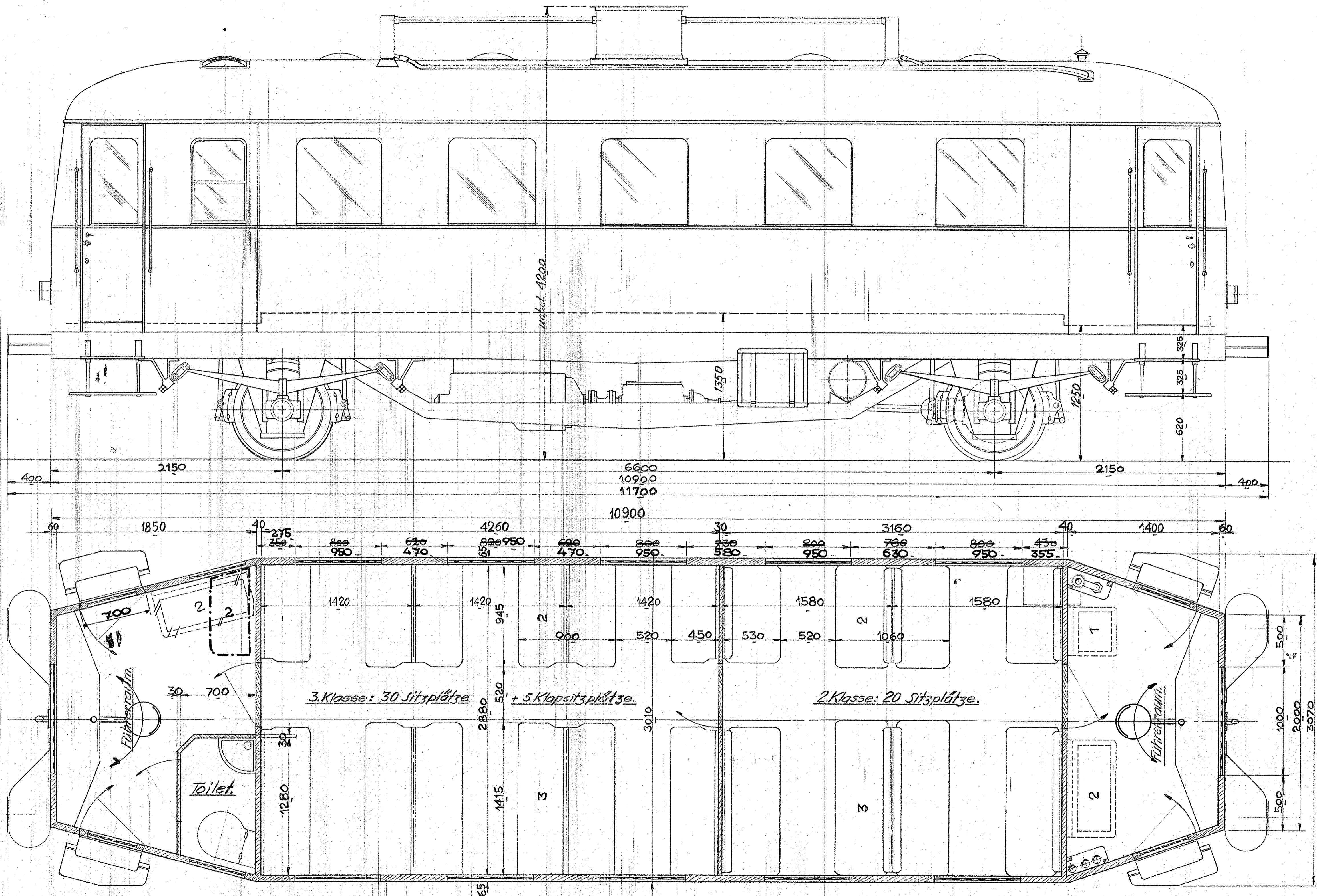
Triebwagen - leichte Type. 50 Sitzplätze. Maßstab 1:20.
