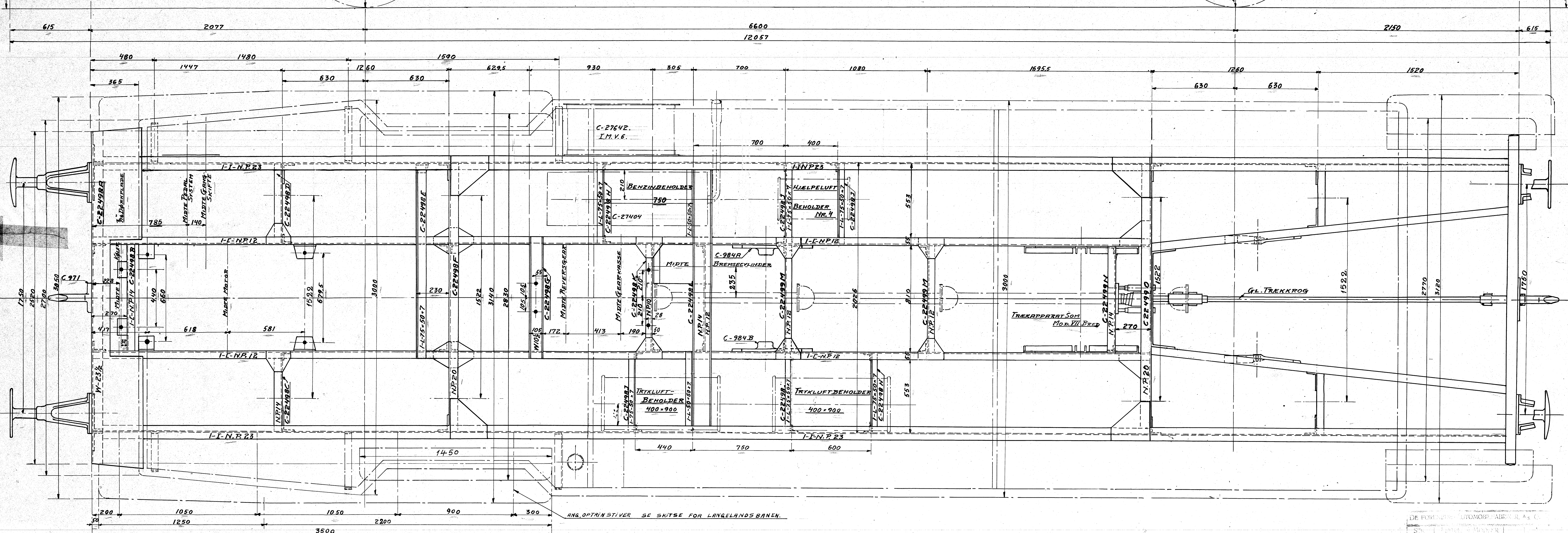
MONTAGETEGNING FOR MOTORVOGN. - LANGE LANDS BANEN. SKALA 1:10.
