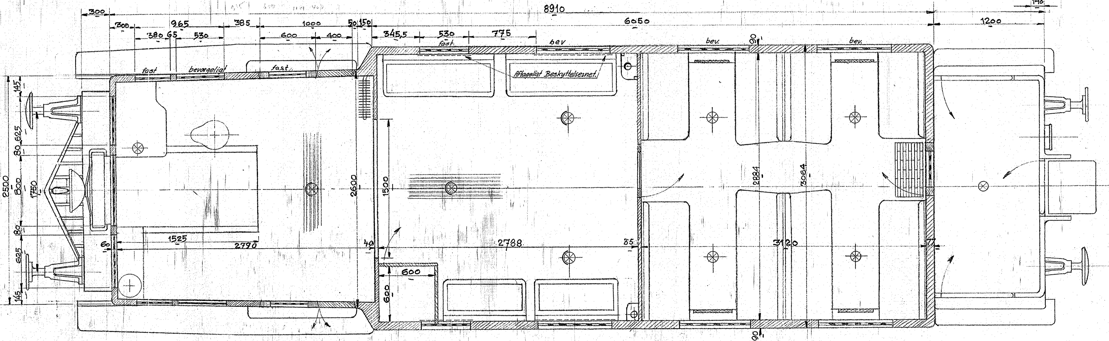
Ombygning af Personvogn til Motorvogn - 30 Siddepladser.
