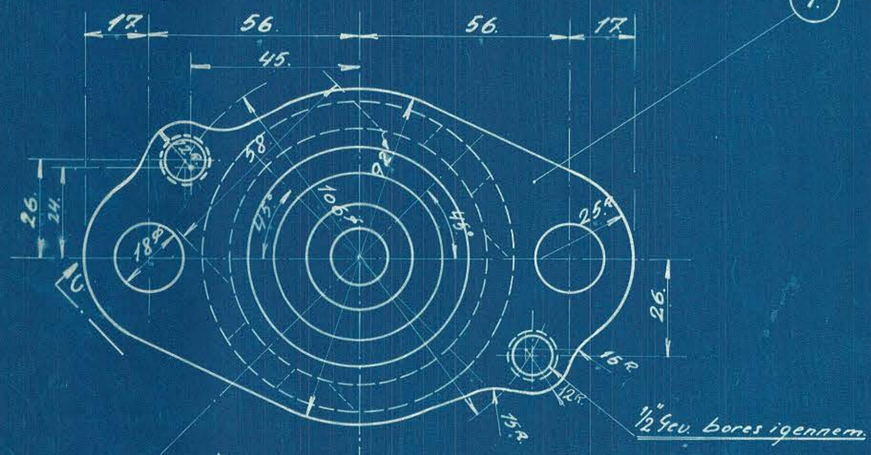
Venstre Ventilhus
