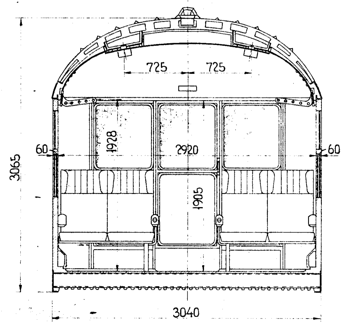
Snit A-A.
