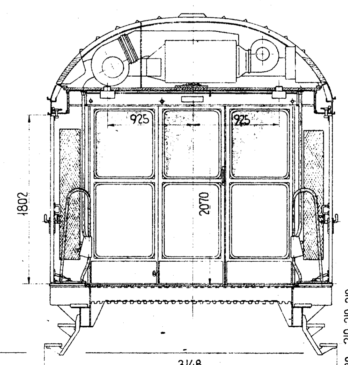
Snit B-B.
