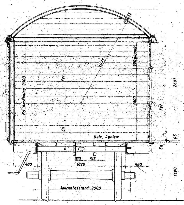
Snit c-d
