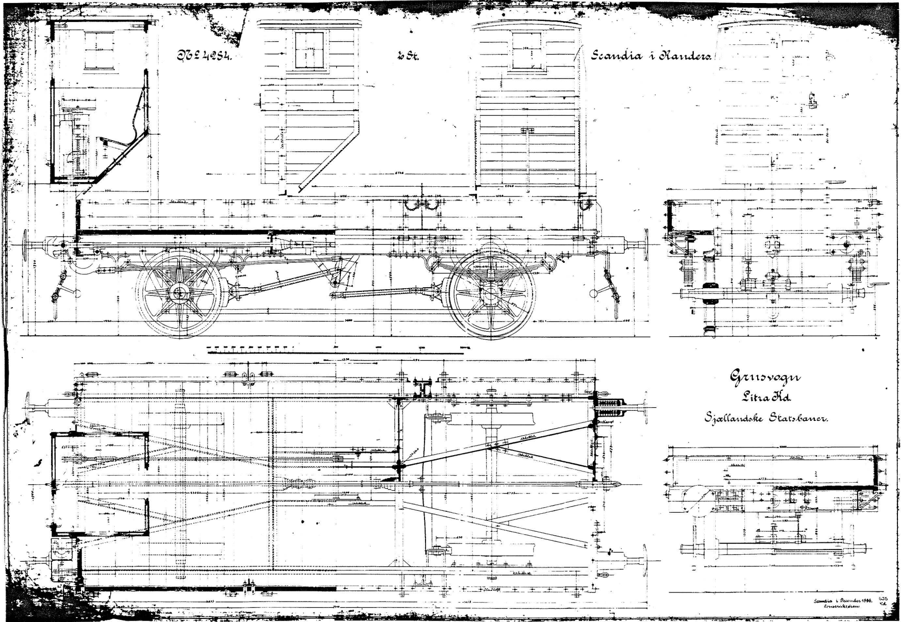
DSB TE 8881-8887 ex PA 6281-6287 ex SJS Ob 1701-1707 (1886) 1:45
