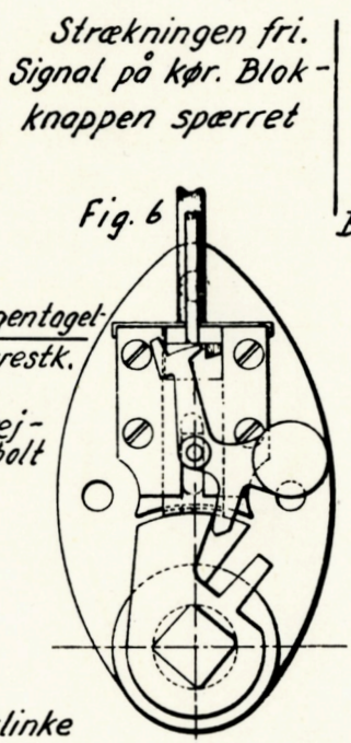
Fig. b. Udkørselslinieblokspærre.
