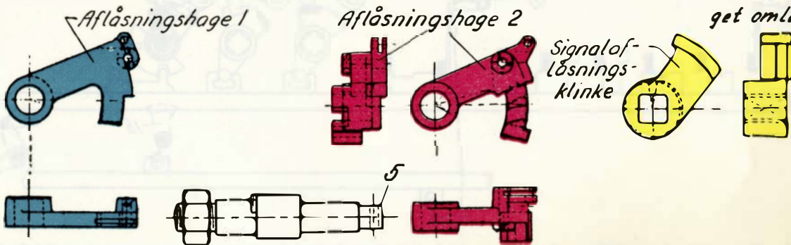
Fig. 0707. Togvejsfastlægningspærre med to stænger, nemlig forlænget blokstang og forlænget trykstang (enheststypen).
