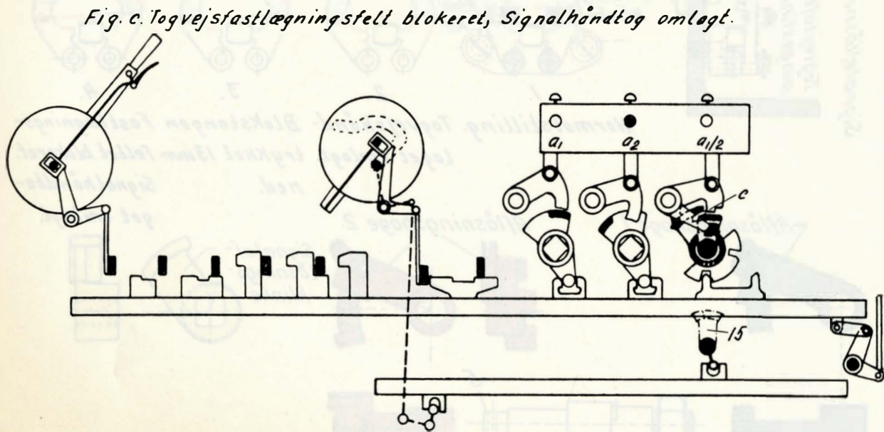
Fig. 0706. Skematisk fremstilling af afhængigheden mellem togvejsfastlægningspærre og togvejshåndtag samt signalhåndtag m. v. (enhedstypen).
