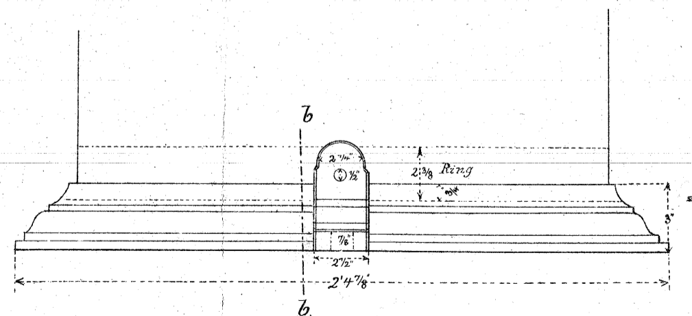
Snit b-b
