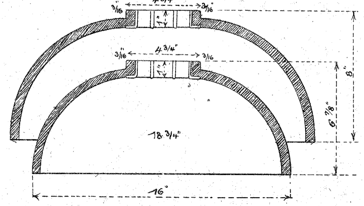
Klokkeskaale
