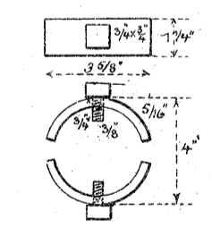
Halbringe
