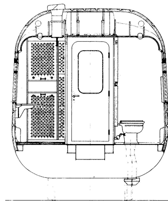
Schnitt P-P
