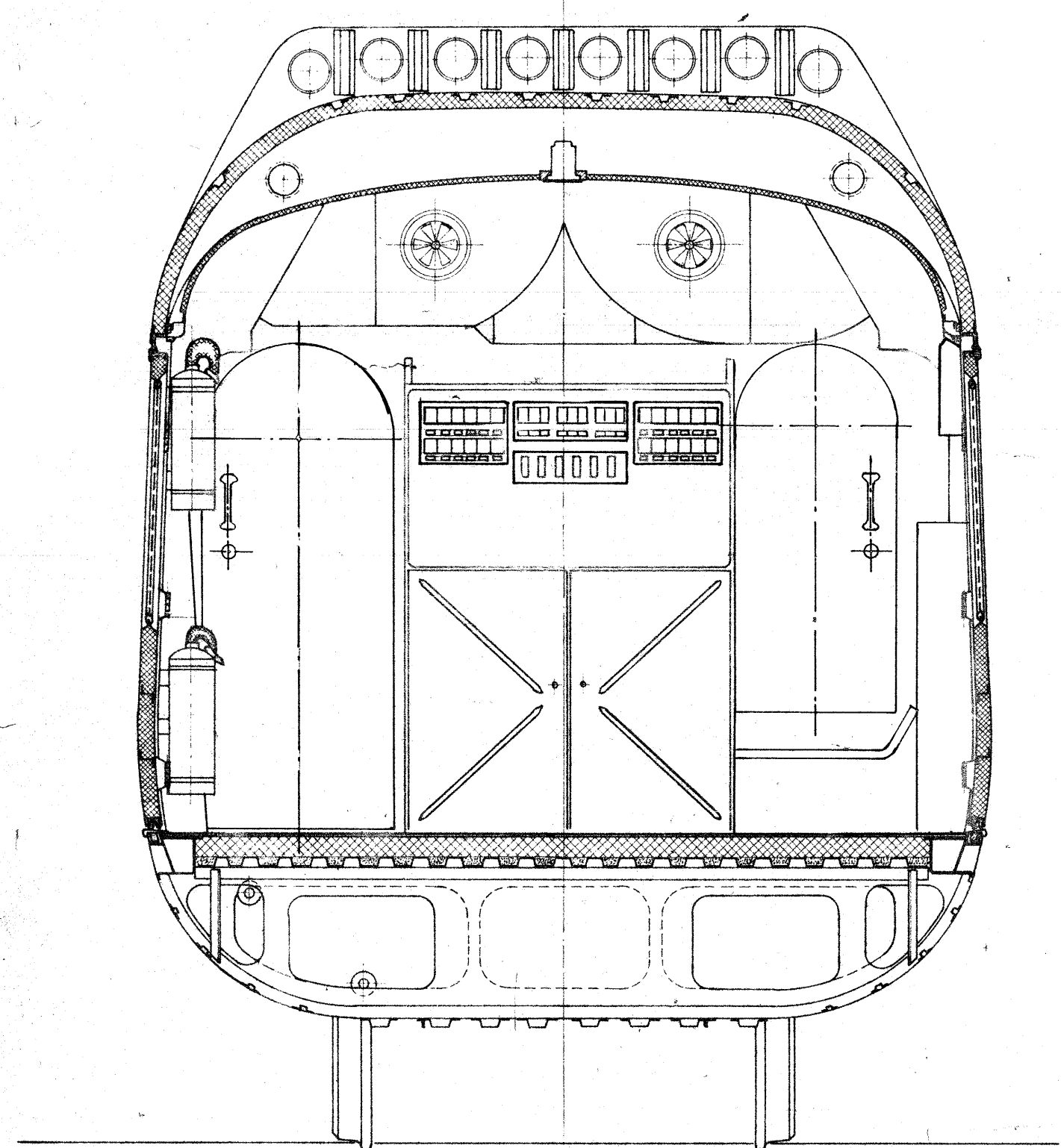
Schnitt H-H
