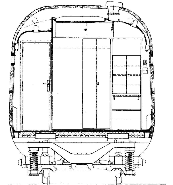
Schnitt M-M
