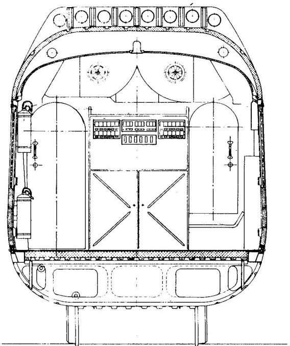
Schnitt H-H
