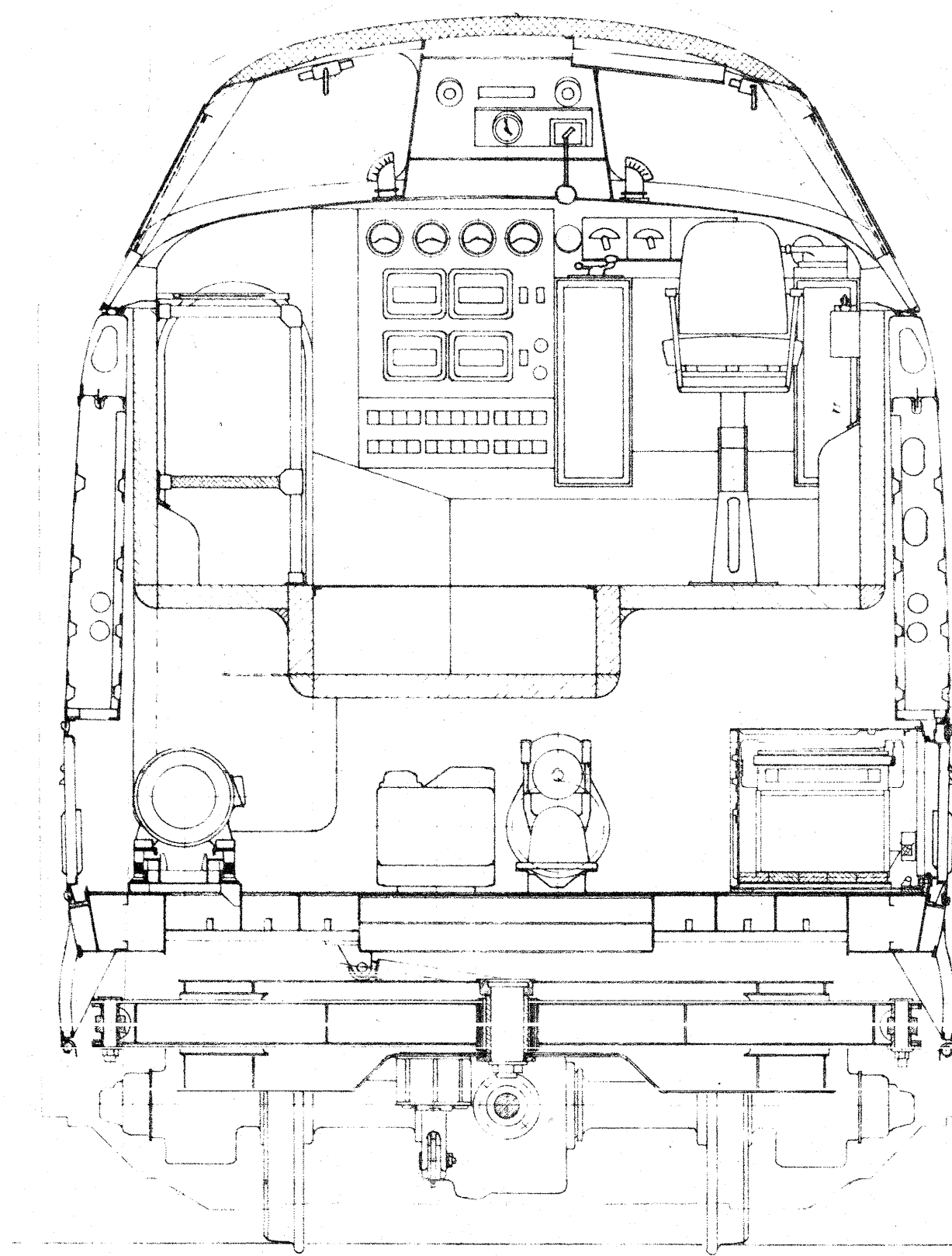
Schnitt G-G
