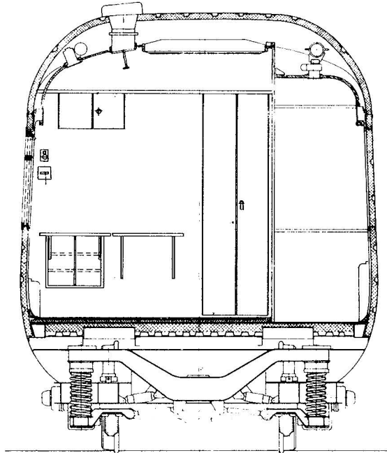
Schnitt L-L
