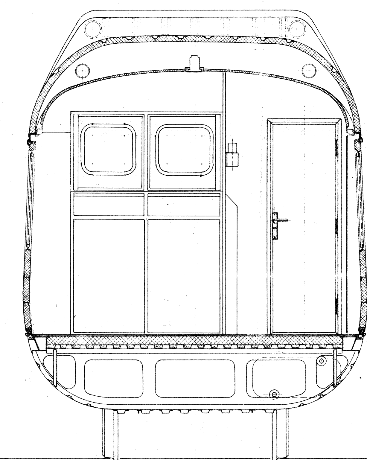
Schnitt J - J
