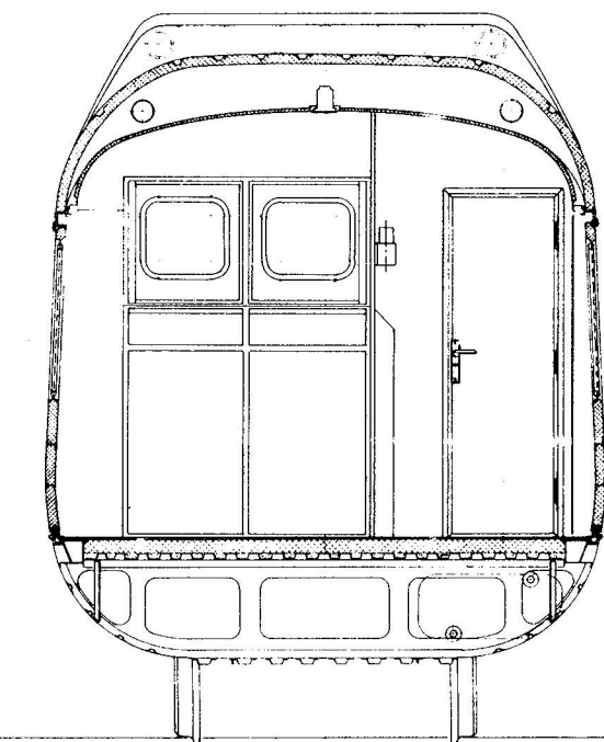
Schnitt J-J
