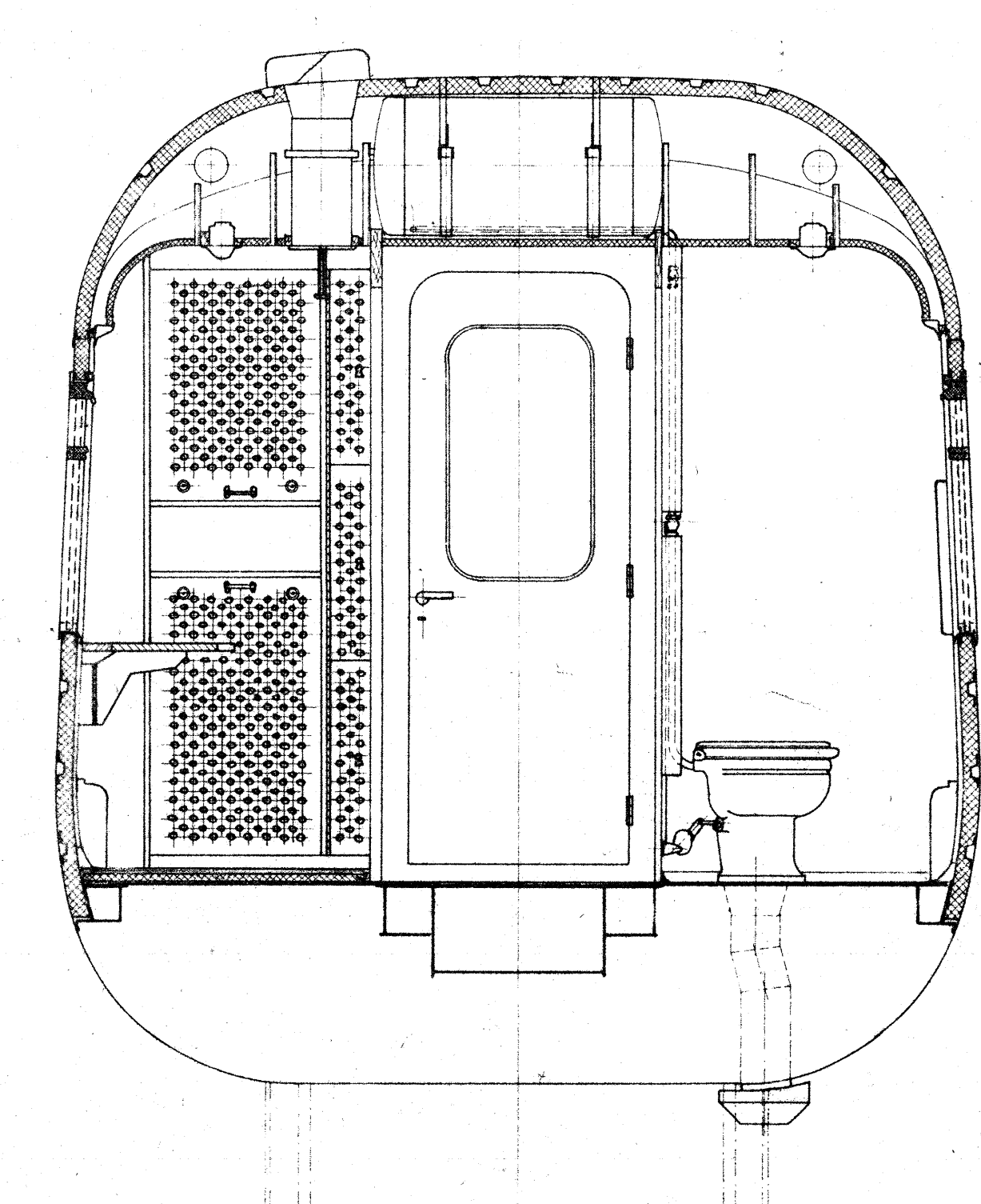
Schnitt P - P .
