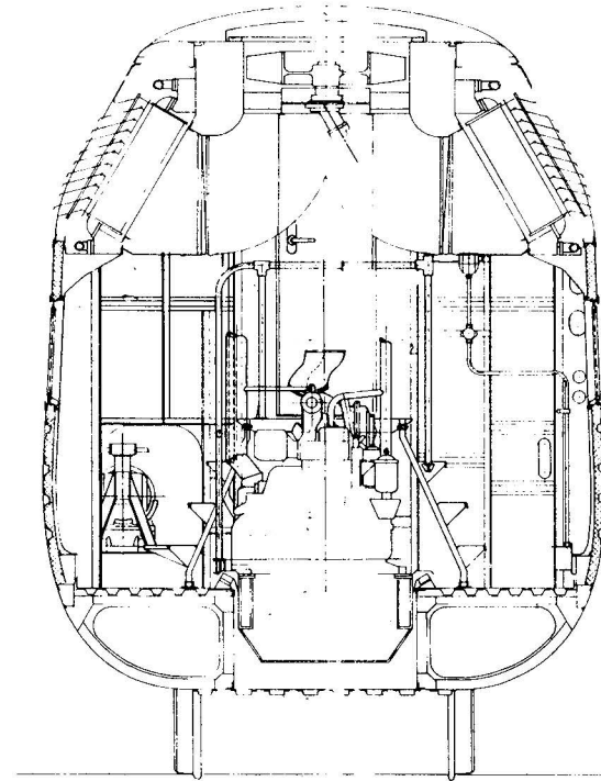
Schnitt E-E
