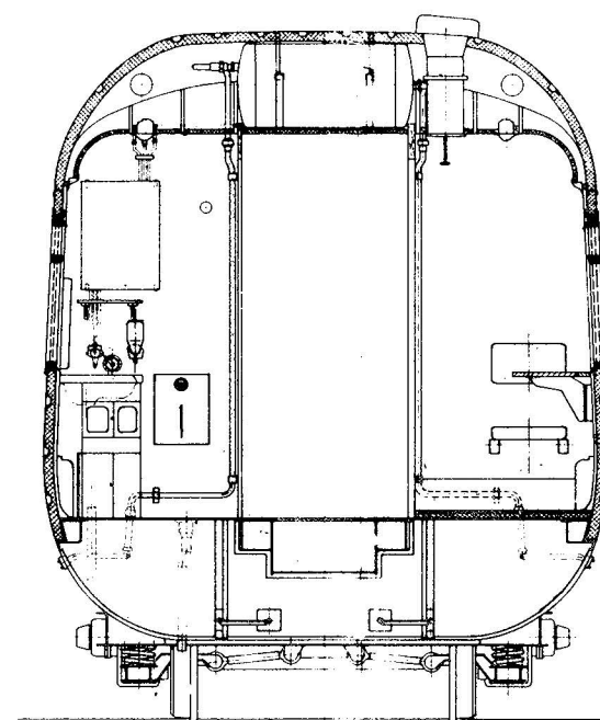
Schnitt Q-Q
