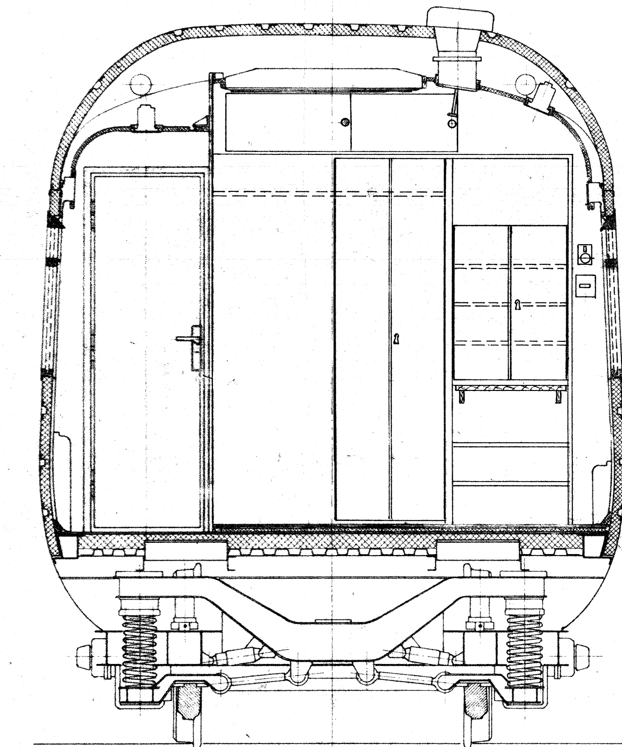
Schnitt M-M
