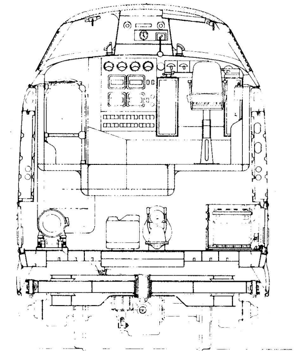
Schnitt G-G
