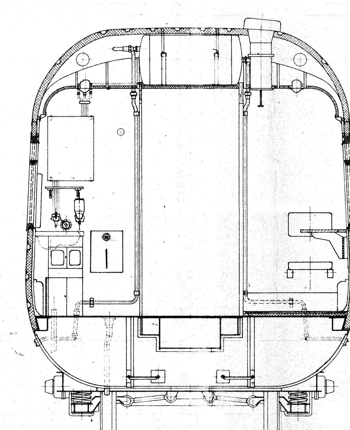
Schnitt Q - Q
