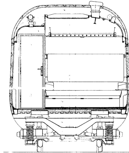
Schnitt K-K
