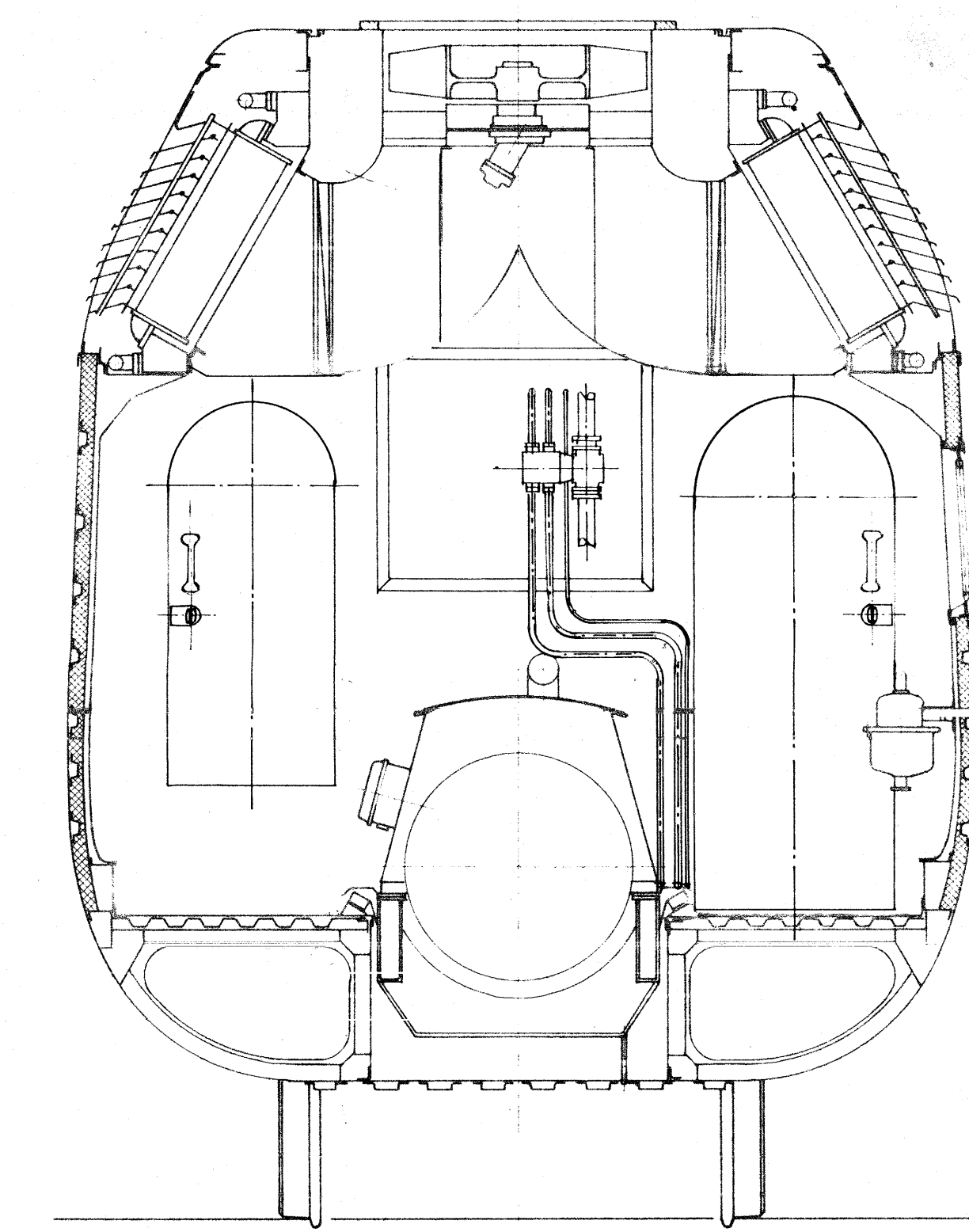
Schnitt F-F
