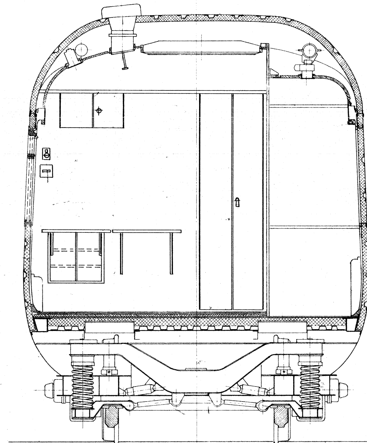
Schnitt L-L
