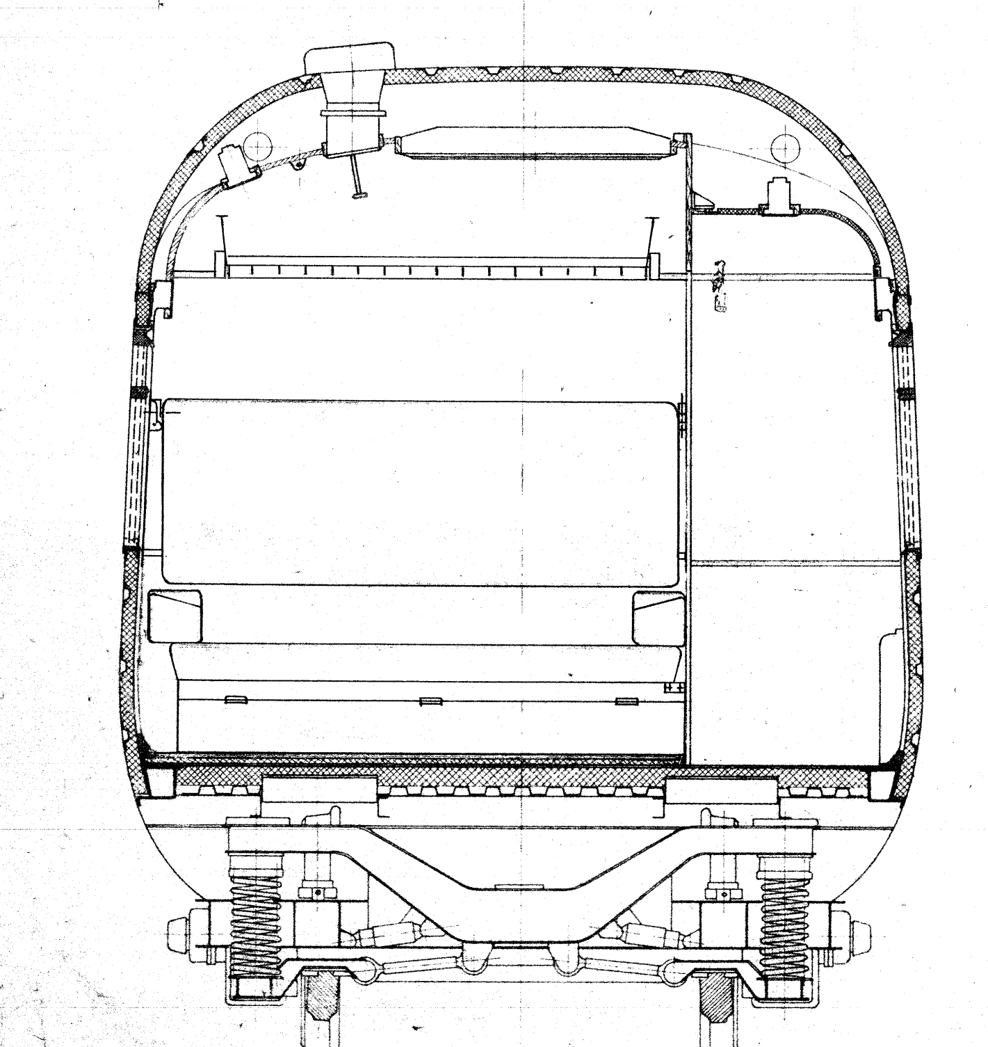
Schnitt N-N
