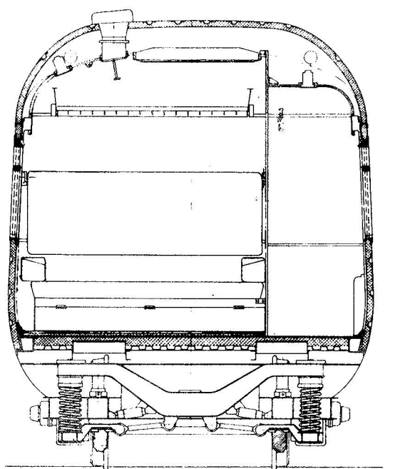
Schnitt N-N
