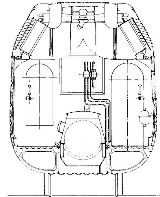
Schnitt F-F
