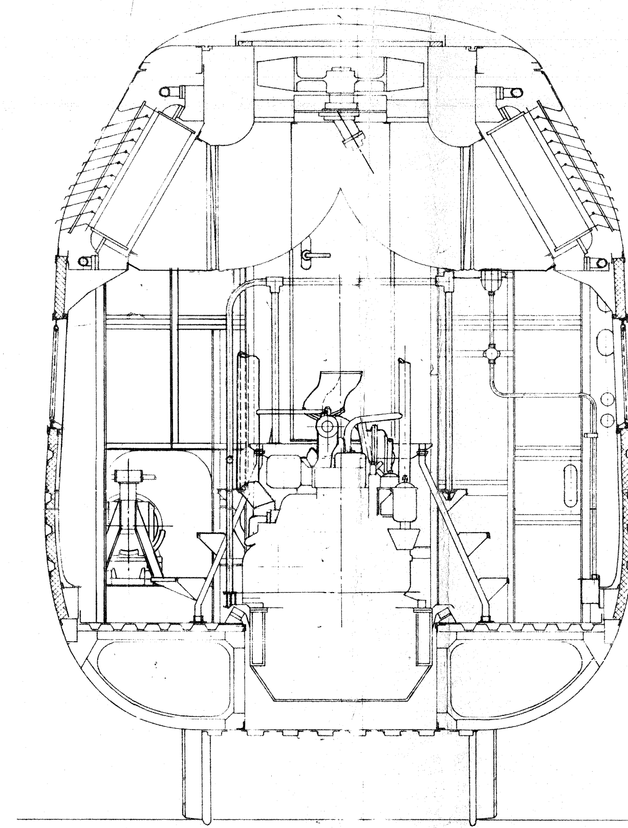
Schnitt E-E
