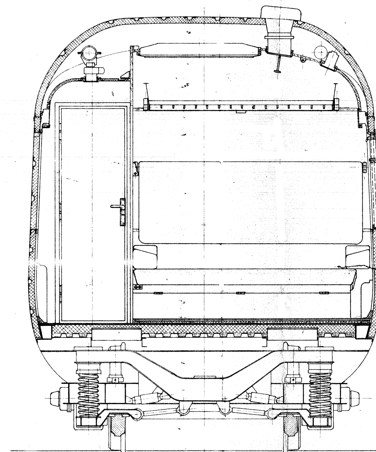
Schnitt K-K
