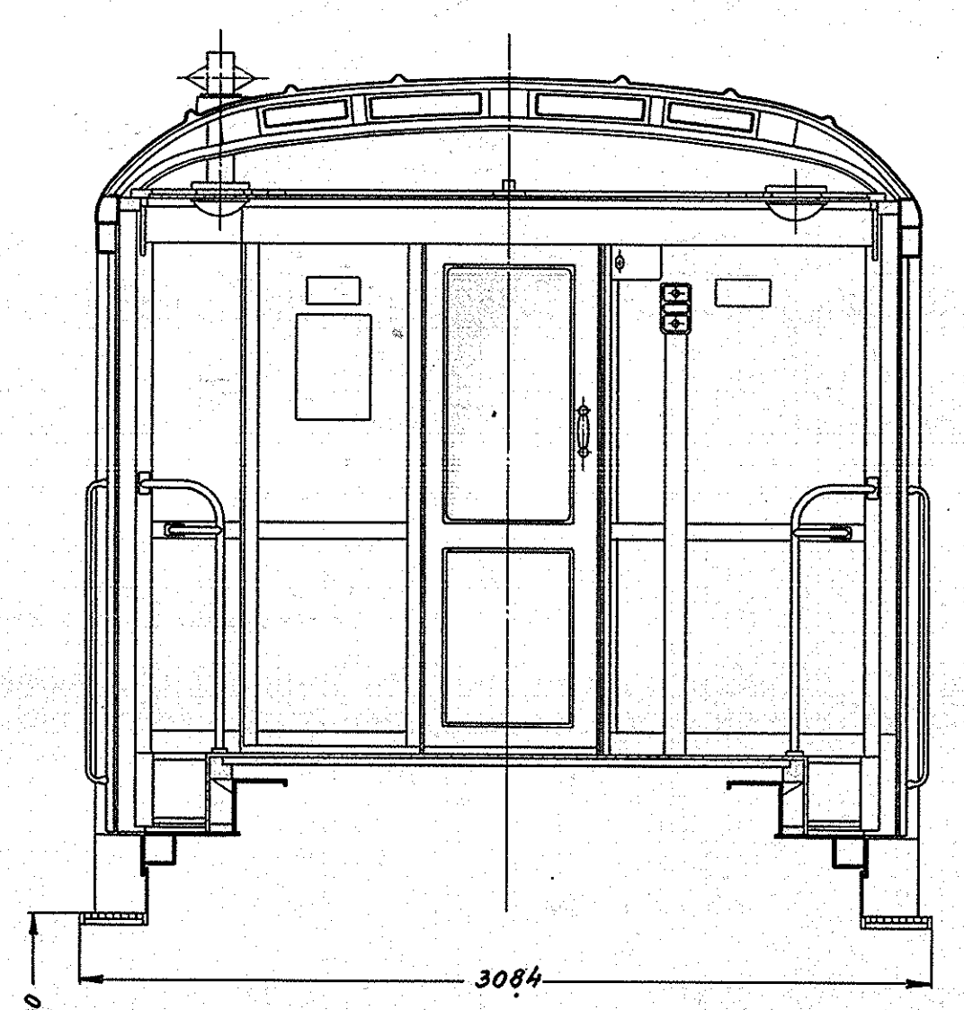
Snit C-C
