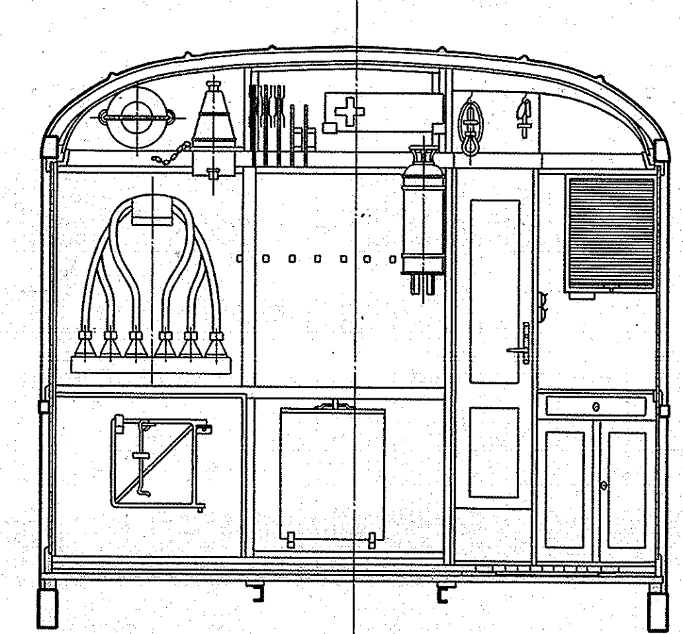
Snit A-A
