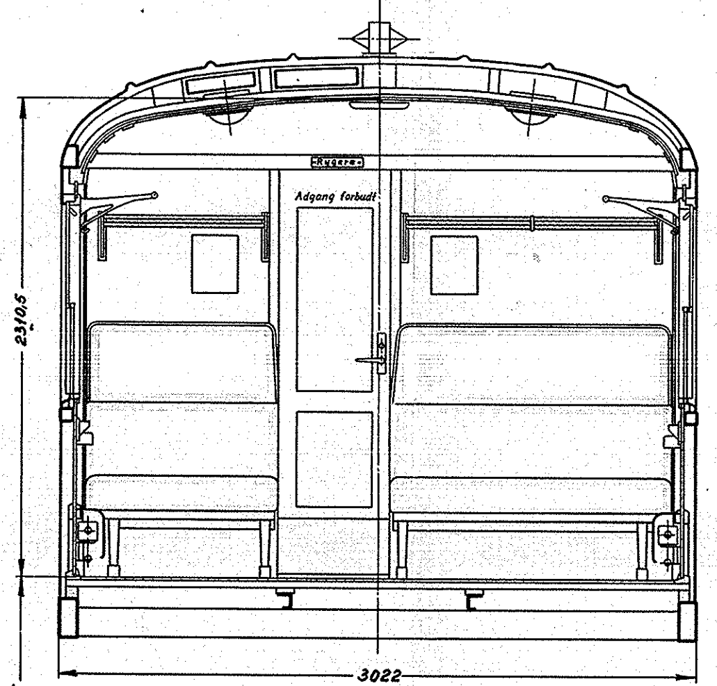
Snit B-B
