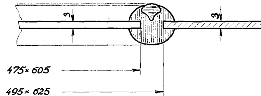
Snit A-A
