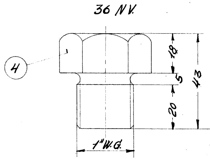
Til udligningsbeholder.
