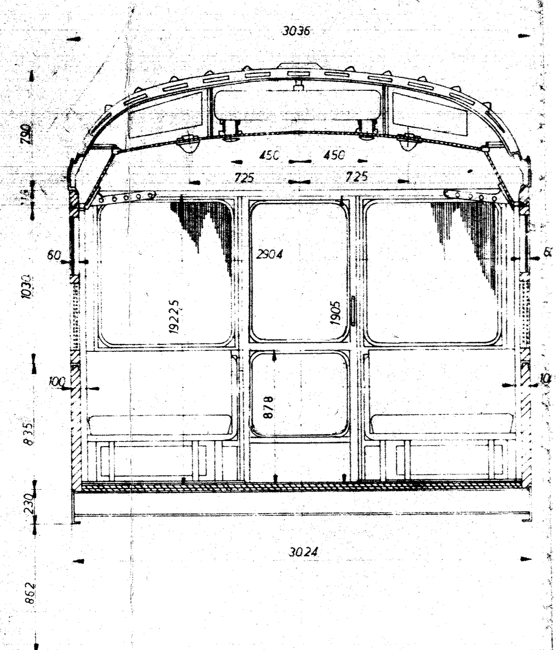
Snit A-A
