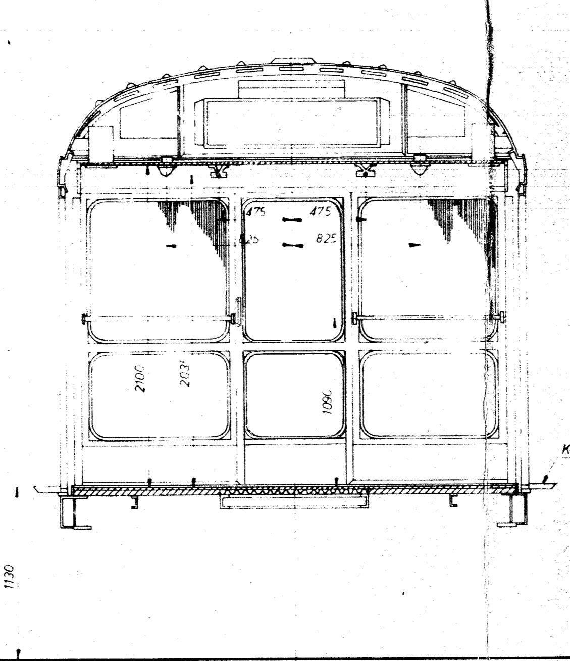
Snit B-B
