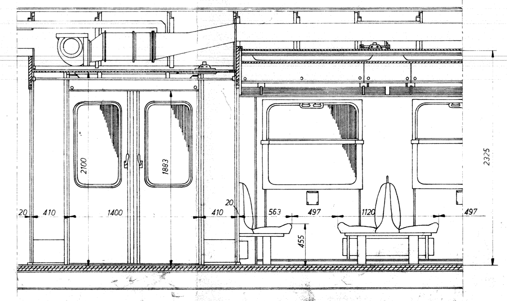
Snit C-C
