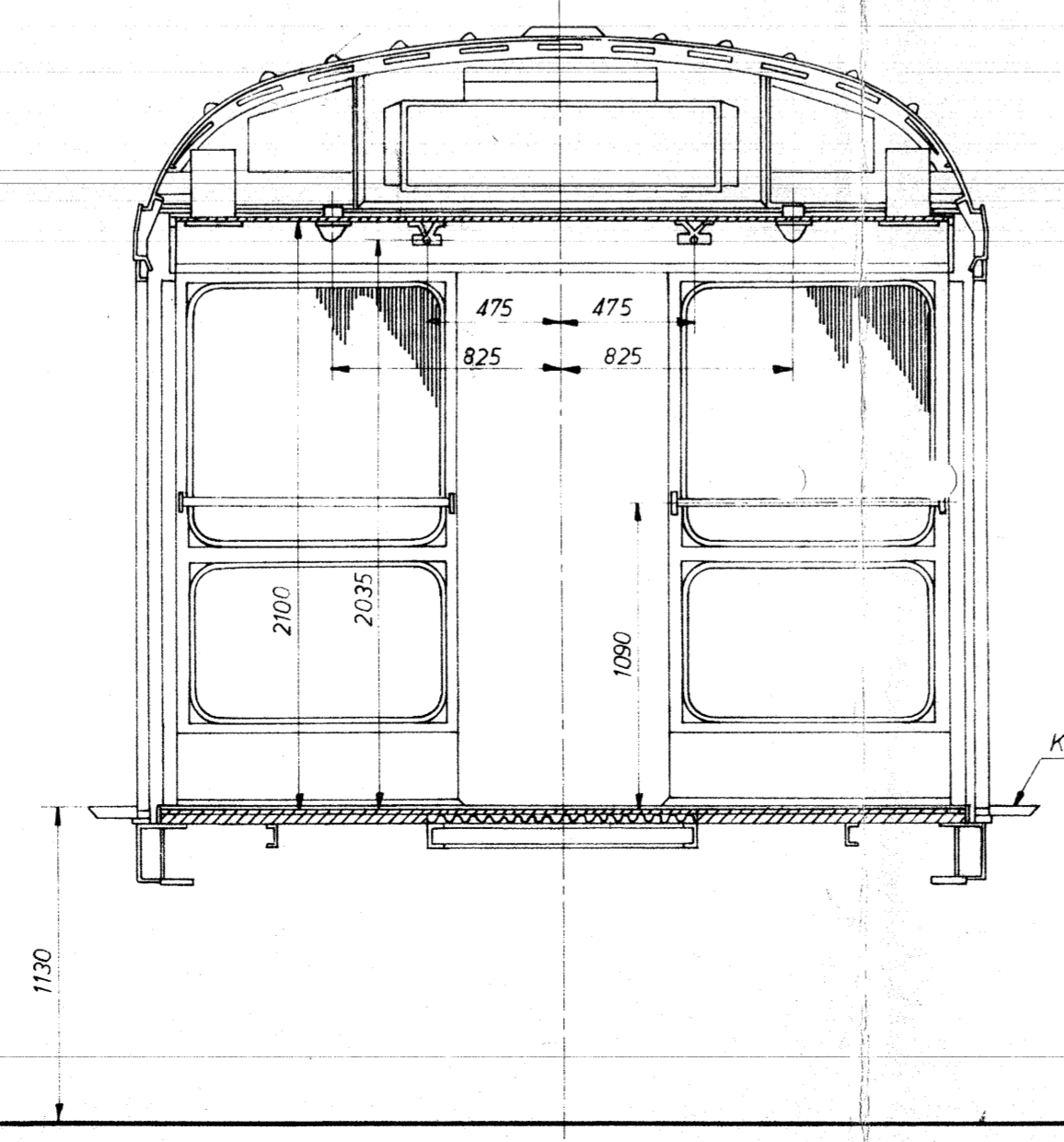
Snit B-B
