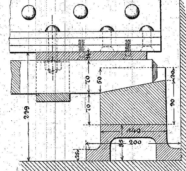
Laaserigel.
