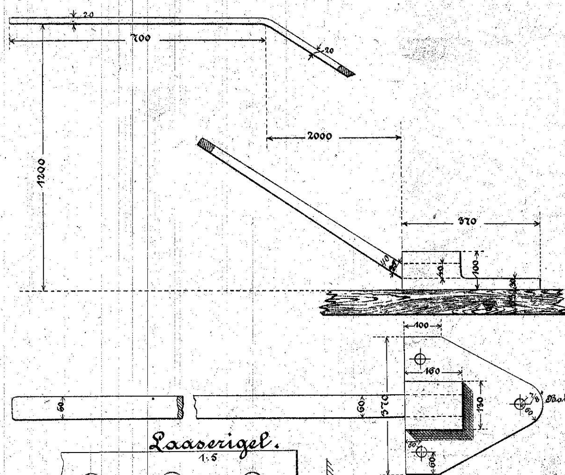
Skydestang.
