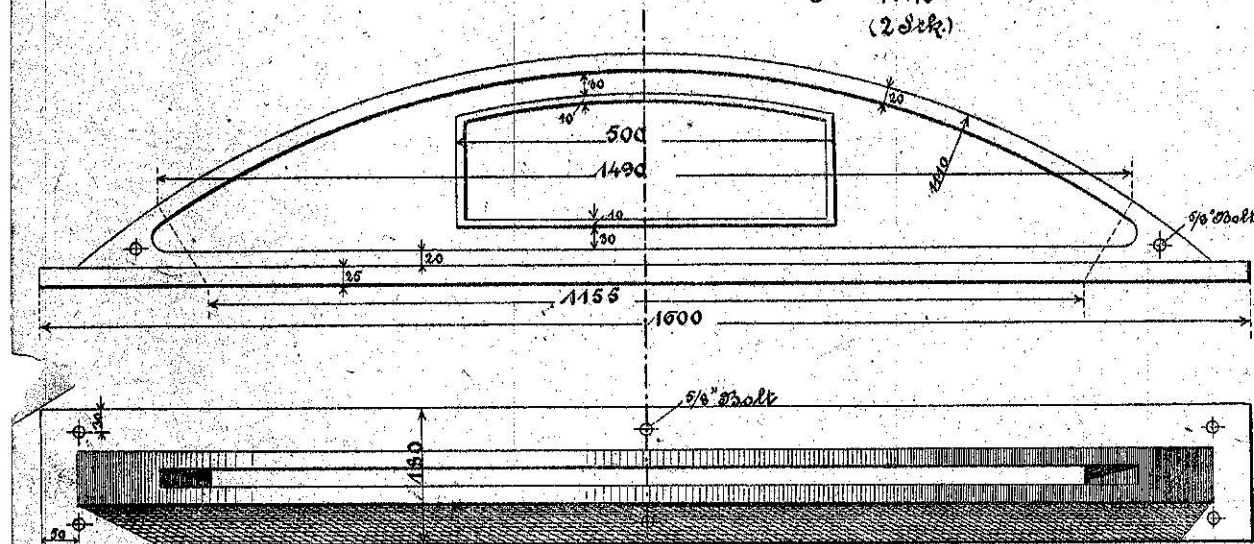
Styreramme.
