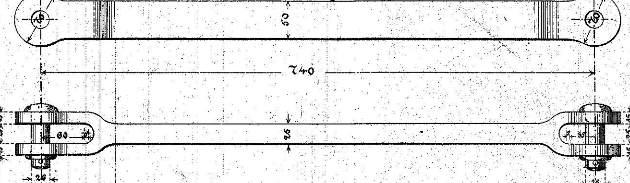
Forbindelsesstang.
