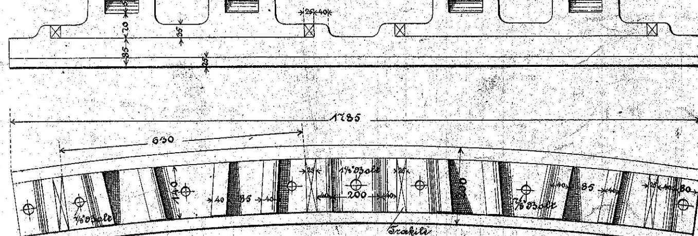
Forbindelsesstang.
