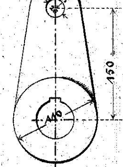
Krumtap.
