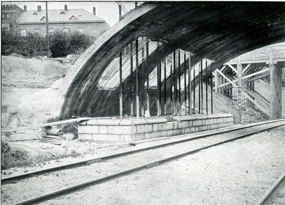
Viadukt ved Ingeniørkasernen under Ombygning
