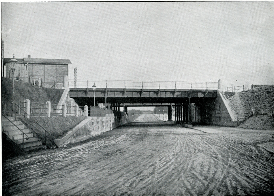
Viadukt over St. Tuborgvej
