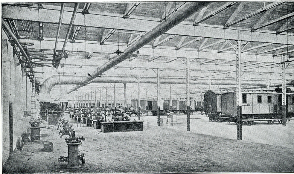
Vognreparationsværksted
