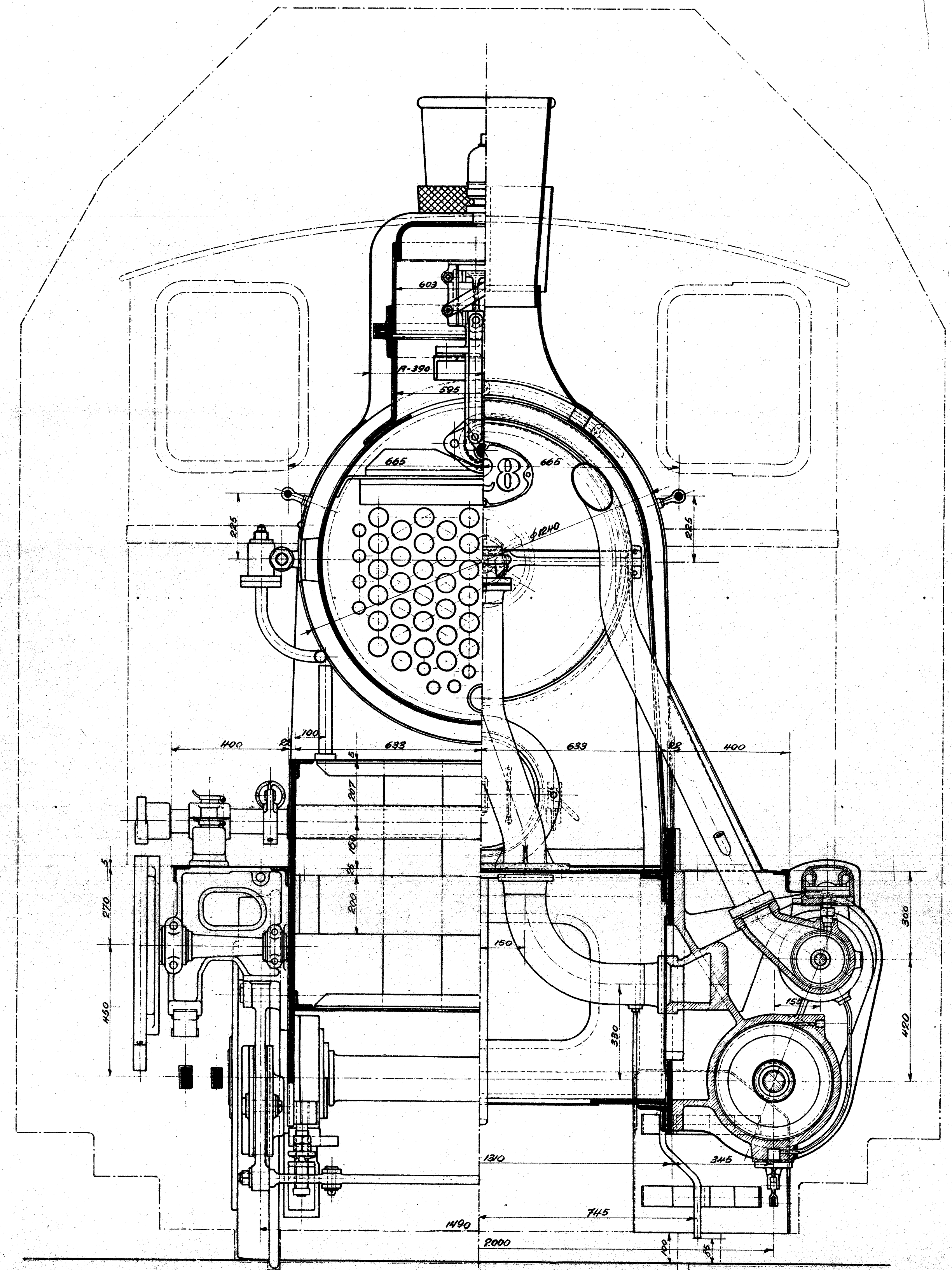
1:10 sand Skærelse.
