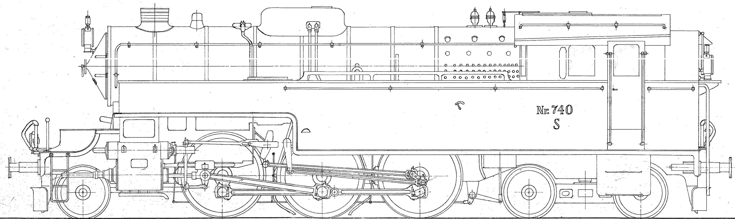
Uden Røgplader og stor Kulkasse. Fødevandspumpe ikke vist, ingen Trykluftbremse.
